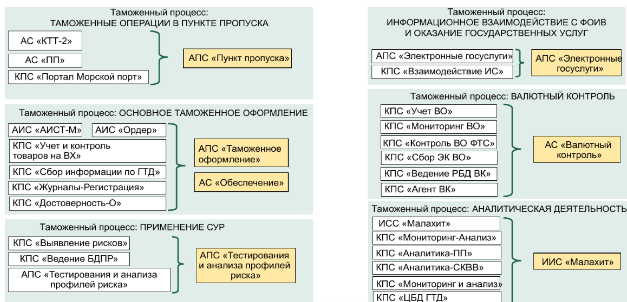
Рис. 5. Изменение архитектуры ЕАИС таможенных органов
