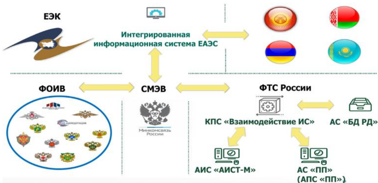
Рис. 6. Организация Интегрированной информационной системы ЕАЭС
