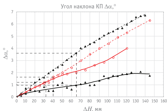
Рис. 11. Диаграмма зависимости угла наклона контактного провода от высоты его подъема: штриховая линия — ветровая нагрузка отсутствует; сплошная линия — при P_{\text{в}} = 250 \text{ Н} ; —○— фиксатор типовой КС-109; —△— фиксатор двойной гибкий
