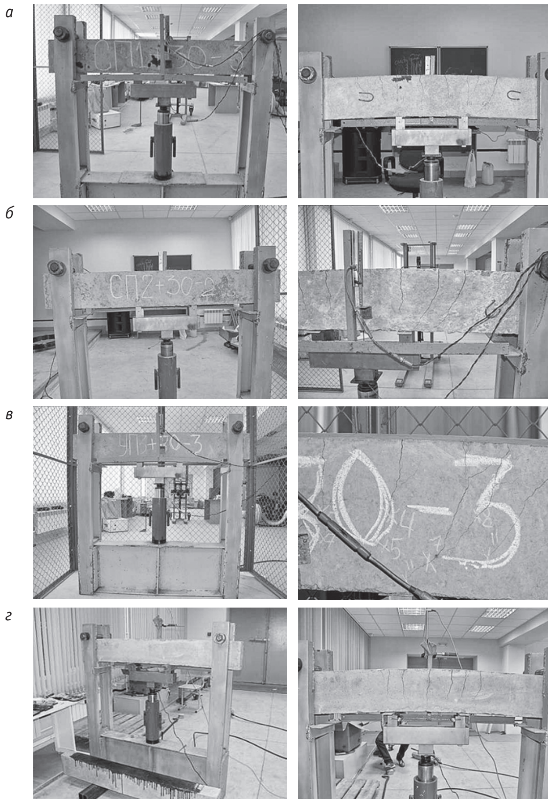
Рис. 4. Вид образцов до и после испытания на прочность: а — серия СП1; б — серия СП2; в — серия УП; г — серия А
