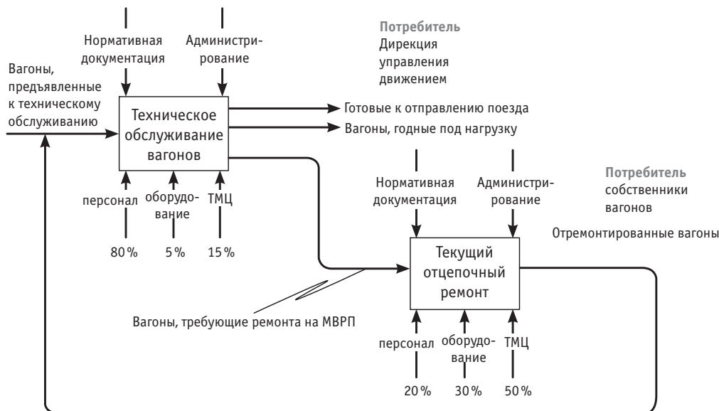
Рис. 1. Модель основных процессов эксплуатационного вагонного депо
