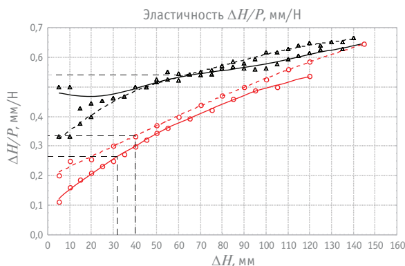
Рис. 12. Диаграмма зависимости эластичности контактной подвески в точке фиксации от высоты подъема контактного провода: штриховая линия — ветровая нагрузка отсутствует; сплошная линия — при P_{\text{в}} = 250 \text{ Н} ; —○— фиксатор типовой КС-109; —△— фиксатор двойной гибкий
