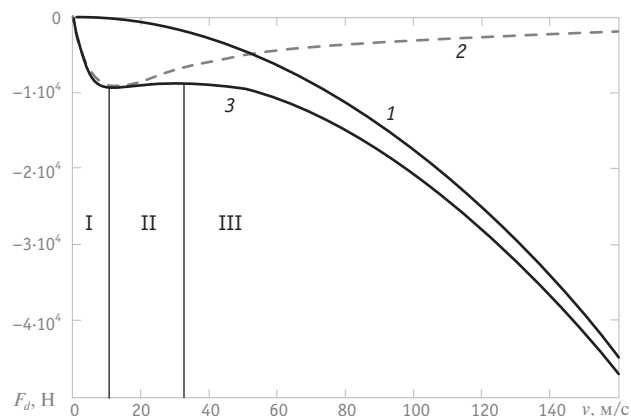
Рис. 3. Зависимость сопротивления движению от скорости:
