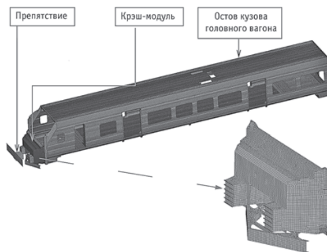
Рис. 4. Конечно-элементная модель головного вагона
