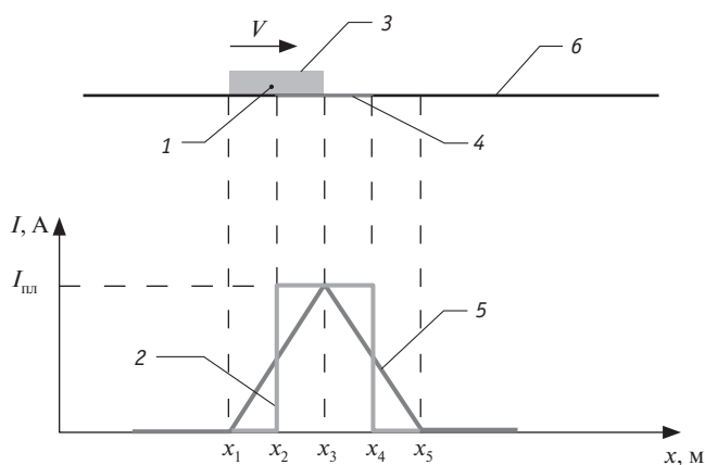
Рис. 1. Расчетная схема для определения тока через ЭКП:
