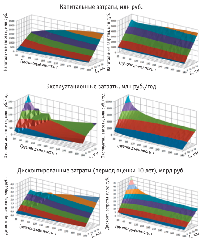
Рис. 1. Результаты расчета технико-экономических показателей транспортирования горной массы карьерными автосамосвалами различной грузоподъемности для вариантов с годовым объемом перевозок 1 млн т (слева) и 40 млн т (справа)
