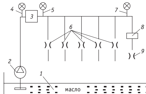
Рис. 1. Функциональная схема системы смазки ДВС:
