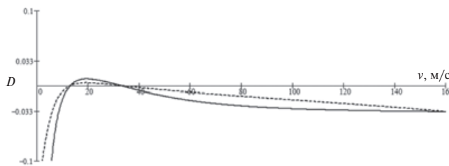
Рис. 13. Скорость изменения энергии колебаний в зависимости от скорости вагона:
