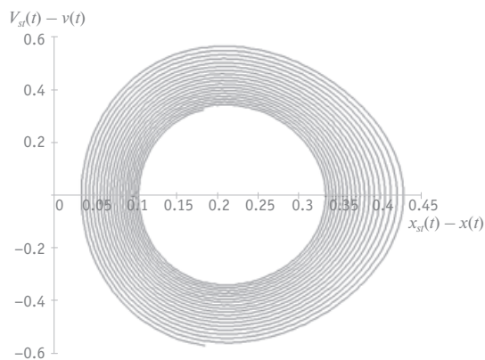
Рис. 5. Фазовая траектория при входе в синхронизм ( v_{st} = 160 м/с)
