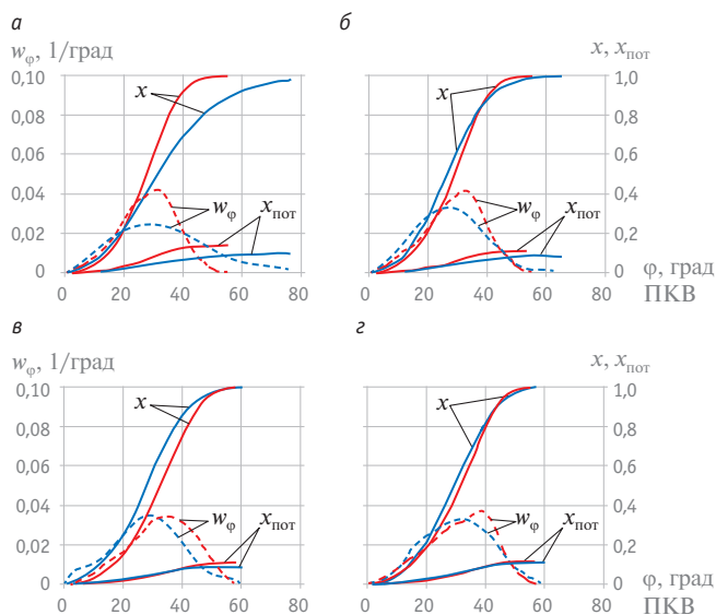
Рис. 3. Интегральные и дифференциальные характеристики выгорания топлива ( n = 2000 \text{ мин}^{-1} ): а — p_e = 0,35 МПа; б — p_e = 0,47 МПа; в — p_e = 0,58 МПа; г — p_e = 0,67 МПа; — при КРМ; — при СРМ
