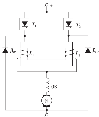
Рис. 1. Принципиальная схема двухфазного тиристорного преобразователя с разделяющим дросселем на общем магнитопроводе:
