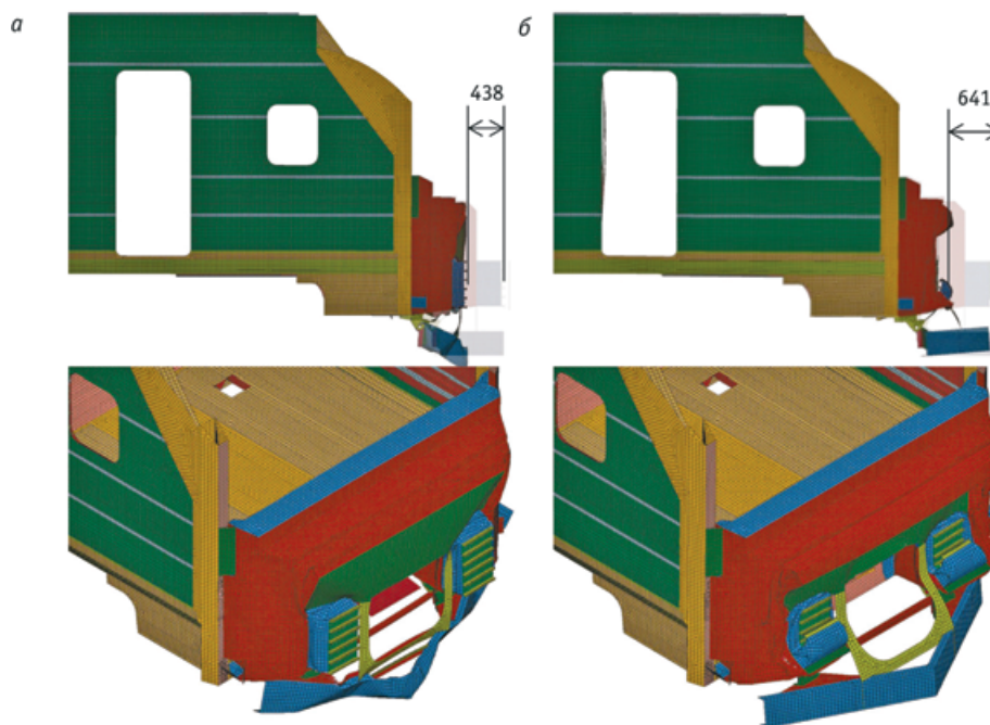
Рис. 5. Разрушение крэш-модуля после столкновения:
