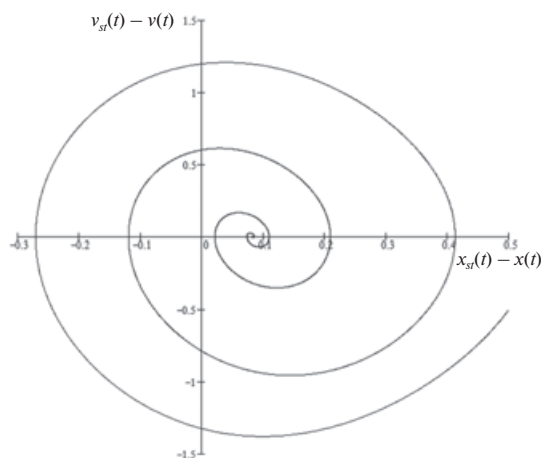
Рис. 14. Фазовая траектория при использовании обратной связи по скорости ( k_0 = 0, 1 )
