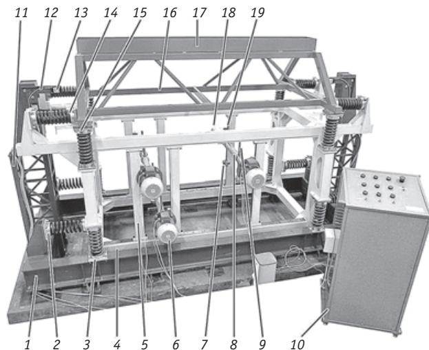
Рис. 3. Учебно-лабораторный комплекс ДВМ-014:
