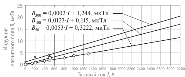
Рис. 5. Зависимость индукции магнитного поля от тока тяги под шинами 3,3 кВ
