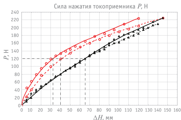
Рис. 10. Диаграмма зависимости силы нажатия токоприемника от высоты подъема контактного провода: штриховая линия — ветровая нагрузка отсутствует; сплошная линия — при P_v = 250 Н; —○— фиксатор типового КС-109; —△— фиксатор двойной гибкий
