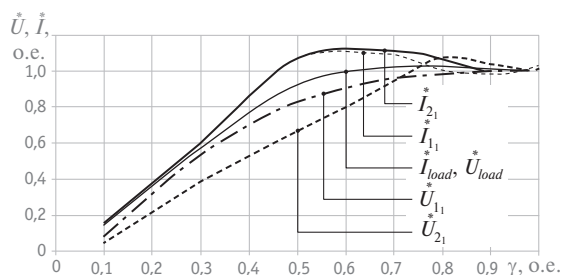
Рис. 3. Регулировочные характеристики ячейки ВИЭ при L_\Phi = 0,1 мГн, C_{\Phi} = 643 мкФ, C_\Phi в соответствии с рис. 2 и неизменном напряжении U_d (зависимости относительных напряжений и токов ячейки ВИЭ от \gamma : для выпрямленных сигналов — постоянная составляющая, для переменных — первая гармоника)
