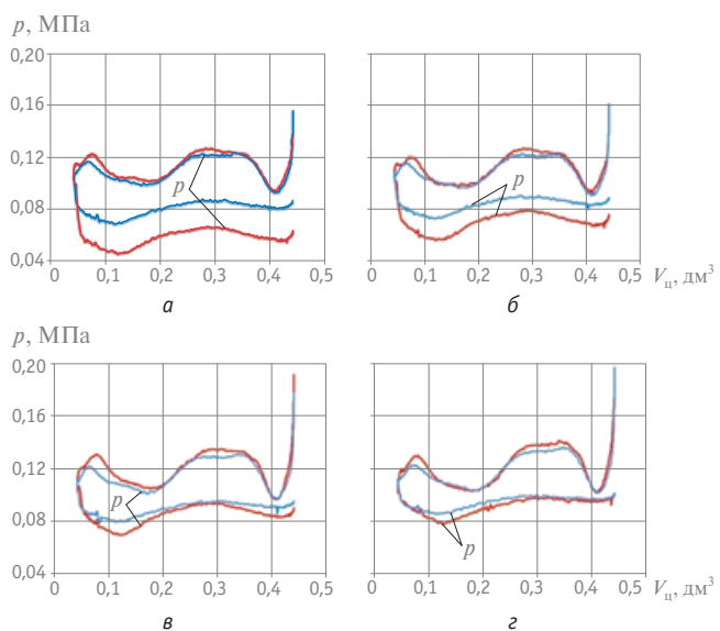
Рис. 4. Изменение давления рабочего тела на тактах впуска и выпуска ( n = 2000 \text{ мин}^{-1} ): а — p_e = 0,35 МПа; б — p_e = 0,47 МПа; в — p_e = 0,58 МПа; г — p_e = 0,67 МПа; — при работе двигателя с КРМ; — при работе с СРМ
