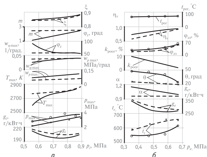
Рис. 1. Зависимость показателей рабочего цикла двигателя от средних индикаторного p_i (а) и эффективного p_e (б) давлений при постоянной частоте вращения коленчатого вала n ( n = 2000 \text{ мин}^{-1} , \Phi_{дз} = \text{var} , k_{роог} = \text{var} , \theta = \text{var} ): — — — КРМ; — — — СРМ
