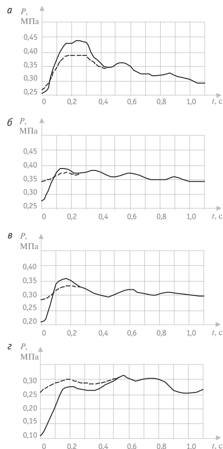
Рис. 2. Изменение величины давления до (пунктирная линия) и после (сплошная) фильтроэлемента при исходном перепаде давления: а — 0,01 МПа; б — 0,065 МПа; в — 0,08 МПа; г — 0,15 МПа
