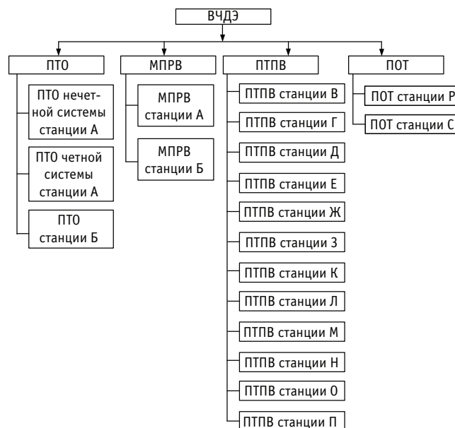
Рис. 2. Структура эксплуатационного вагонного депо (ВЧДЭ)
