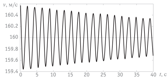
Рис. 4. Колебания скорости при входе в синхронизм ( v_{st} = 160 м/с)
