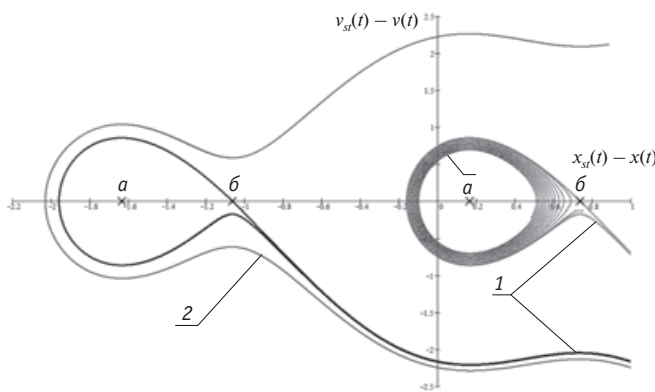
Рис. 6. Фазовые траектории при v_{st} = 160 м/с: 1 — граничные; 2 — расходящаяся; 3 — сходящаяся; а, б — соответственно точки устойчивого и неустойчивого равновесия
