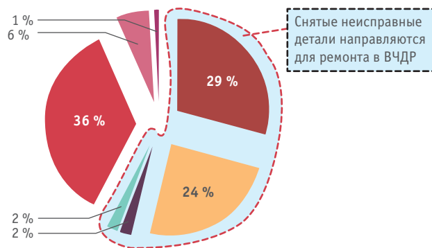
Рис. 3. Причины текущего отцепочного ремонта грузовых вагонов: колесные пары; тележка; тормозное оборудование; автосцепное оборудование; кузовные работы; рама вагона; прочие работы
