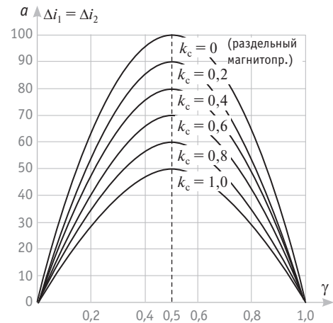
Рис. 4. Зависимость пульсации тока a в разделяющих дросселях от коэффициента заполнения \gamma при различных значениях коэффициента связи K_c
