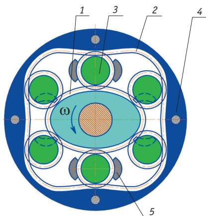
Рис. 1. Планетарная роторная гидромашина (схема M = 2 , N = 4 , K = 6 , P = 8 ) [2]: 1, 2 — центральные колеса с внешними и внутренними зубьями; 3 — сателлиты; 4 — корпус насоса; 5 — каналы подвода и отвода рабочей среды
