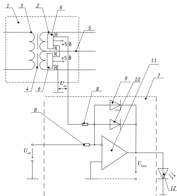
Рис. 2. Устройство сигнализации о наличии асимметрии тягового тока в рельсовых цепях:
