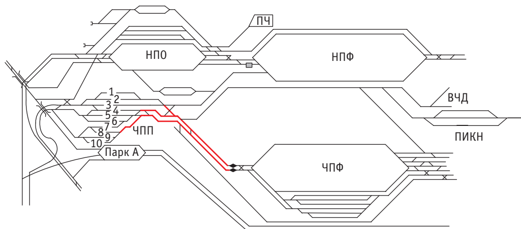
Рис. 4. Маршрут пропуска через сортировочную горку вагонов с коммерческими неисправностями
