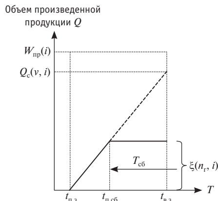
Рис. 3. Графическое представление состояния \varepsilon(n_{исп}, i) = 0 : t_{п.сб} — время появления сбоя; T_{сб} — продолжительность сбоя
