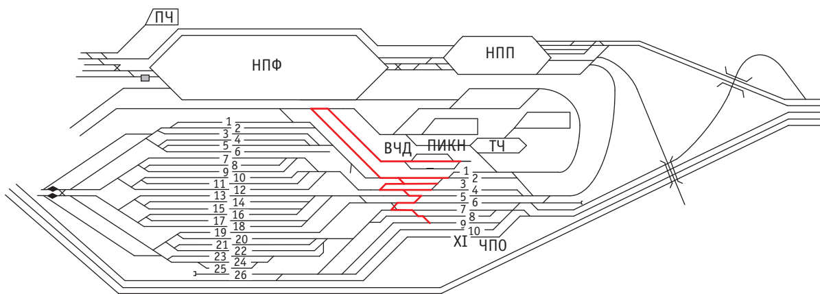
Рис. 9. Схема передвижений в горловине парка отправления при подаче вагонов на ПИКН
