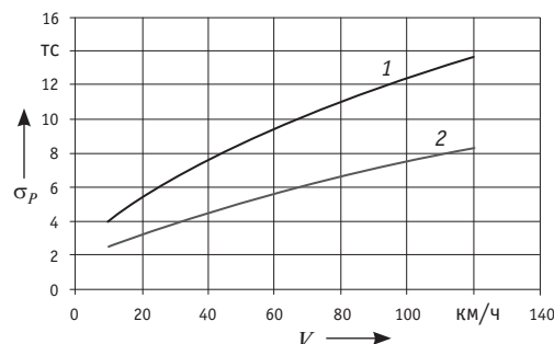
Рис. 7. Среднеквадратическое отклонение динамической добавки давления на рельс:
