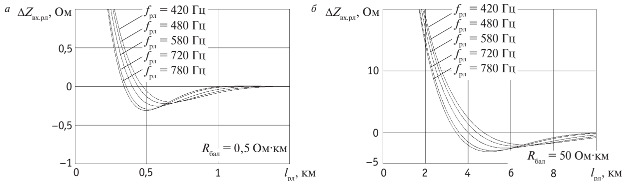
Рис. 5. Зависимость разности сопротивлений короткого замыкания и холостого хода рельсовой линии на частотах ТРЦ от ее длины:
