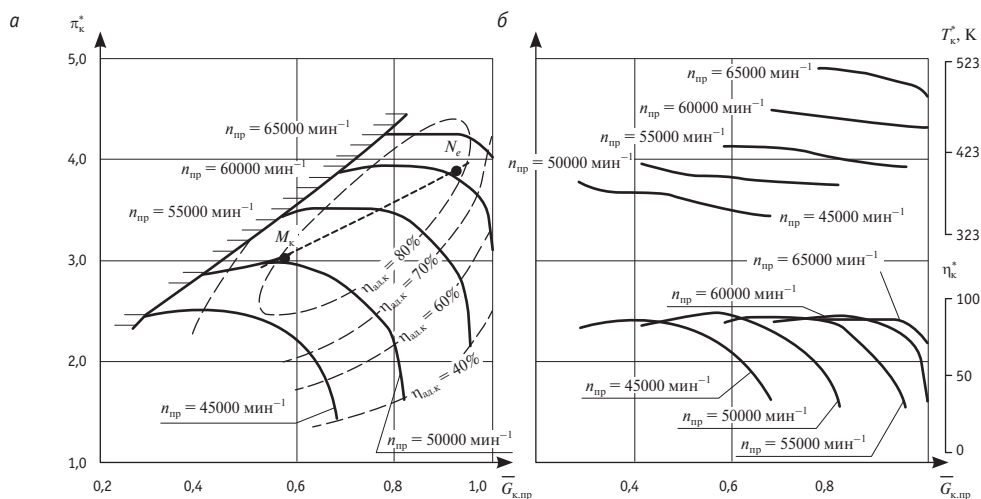
Рис. 4. Изменение основных параметров, характеризующих работу компрессора, в зависимости от относительного приведенного массового расхода воздуха G_{k,пр} :
