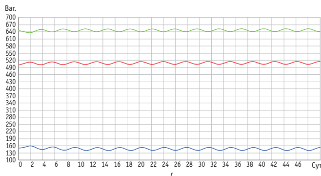
Рис. 7. График динамики изменения количества вагонов на подъездных путях предприятия С: — x(t) — прибыло груженных; — y(t) — прибыло порожних; — z(t) — отправлено груженных/порожних
