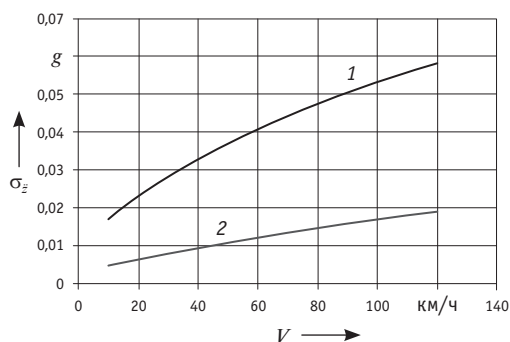
Рис. 5. Среднеквадратическое отклонение ускорения кузова:
