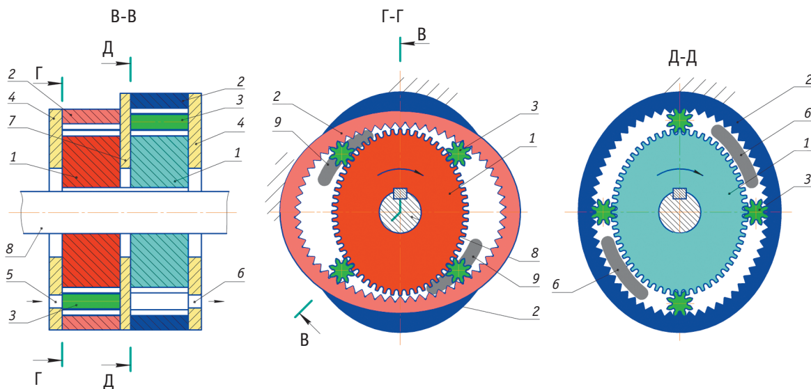
Рис. 2. Роторная гидромашина ( M = 2 , N = 2 , K = 4 ) [7]: 1, 2 — центральные колеса с внешними и внутренними зубьями; 3 — сателлиты; 4, 7 — торцовые перегородки; 5, 6, 9 — каналы подвода и отвода рабочей среды; 8 — вал
