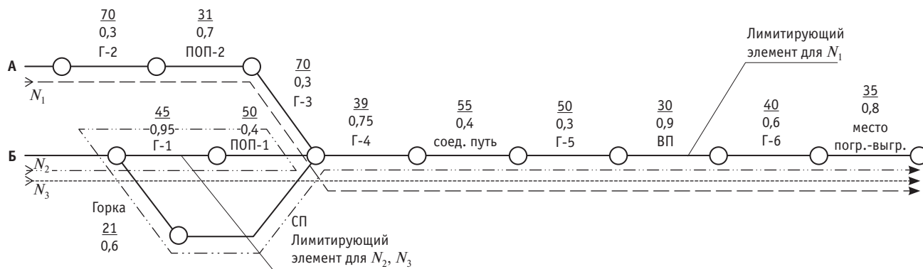
Рис. 1. Схема графа элементов станции примыкания железнодорожного пути общего пользования:
