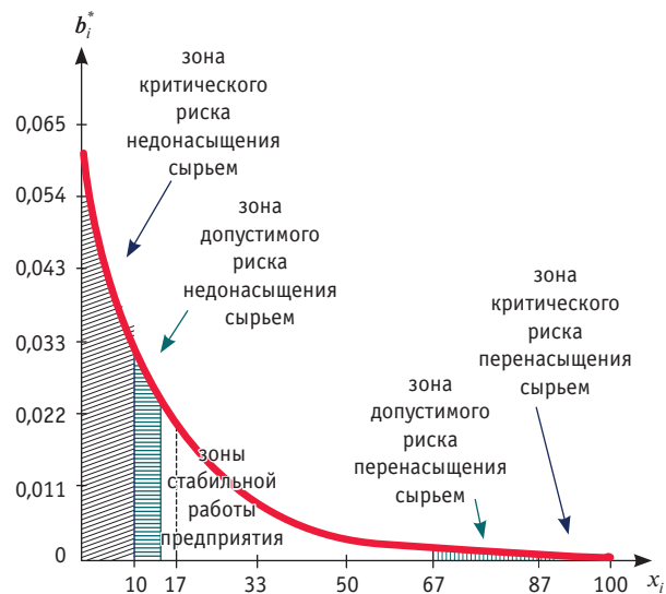
Рис. 3. График плотности и зон риска прибытия груженых вагонов в адрес предприятия G:
