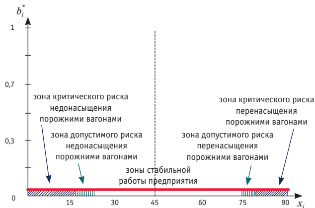
Рис. 6. График плотности и зон риска прибытия порожних вагонов в адрес предприятия D: 0–20, 80–90 — зоны критического риска; 20–25, 75–80 — зоны допустимого риска; 22–45, 45–75 — зоны стабильной работы
