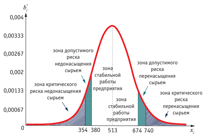
Рис. 1. График плотности и зон риска прибытия груженых вагонов в адрес предприятия С:
