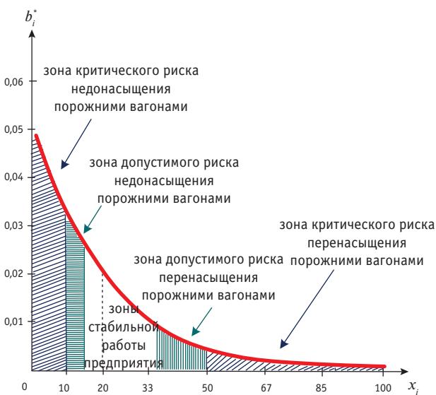
Рис. 4. График плотности и зон риска прибытия порожних вагонов в адрес предприятия G:
