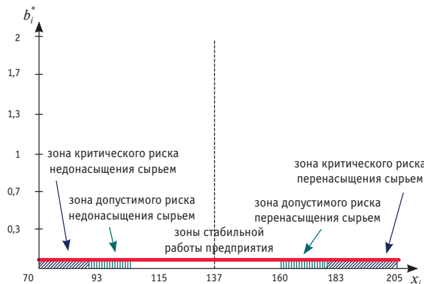
Рис. 5. График плотности и зон риска прибытия груженных вагонов в адрес предприятия D: 70–90, 180–205 — зоны критического риска; 90–105, 160–180 — зоны допустимого риска; 105–137, 137–160 — зоны стабильной работы
