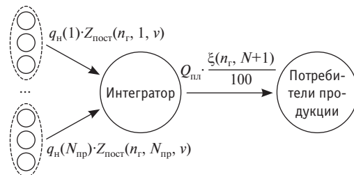
Рис. 5. Графоаналитическое представление производственной цепочки в организационной сети при \varepsilon(n_t, N + 1) = 0 и Z_{пост}(n_t, 1 : N_{пр}, v) < 1
