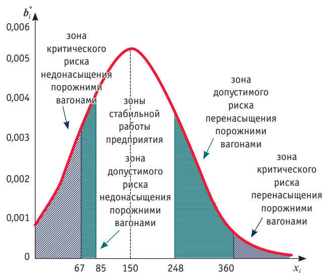
Рис. 2. График плотности и зон риска прибытия порожних вагонов в адрес предприятия С:
