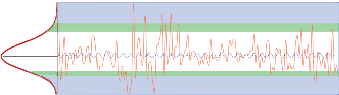
Рис. 8. График сопоставления реальных процессов поступления вагонов с сырьем на предприятие С и результатов численных решений
