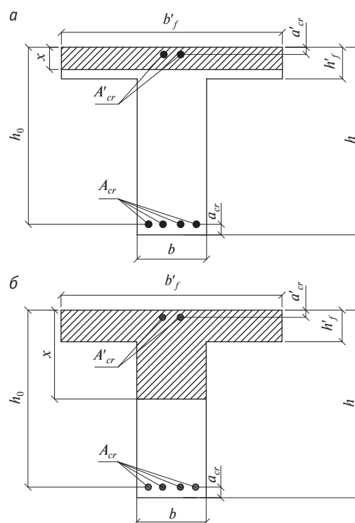
Рис. 2. Расчетное сечение тавровой балки при расположении границы сжатой зоны в плите (а) и в ребре (б)
