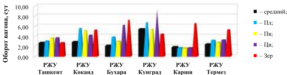
Рисунок 3 – Информация по выполнению оборота вагона по региональным железнодорожным узлам АО «УТЙ» за 2023 г.
