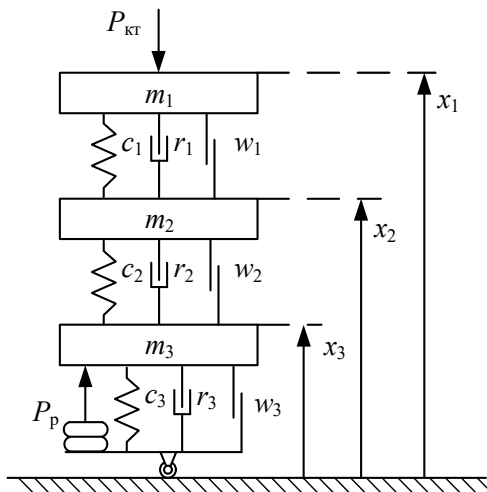
Рисунок 1 – Обобщенная расчетная схема трехмассовой модели токоприемника
