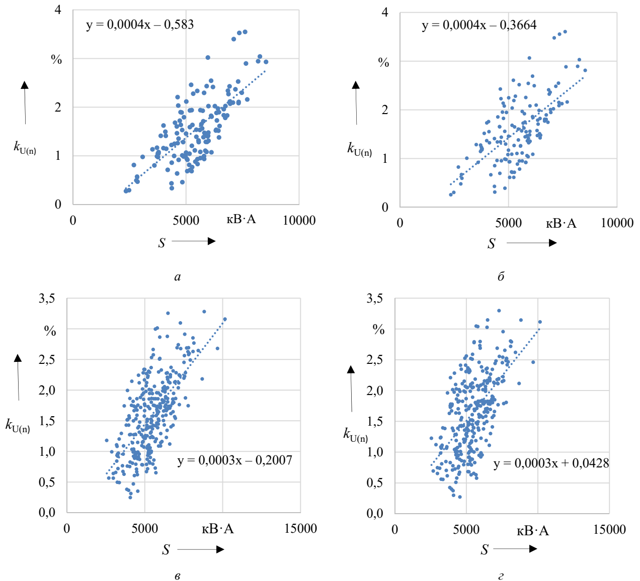
Рисунок 11 – Коэффициенты высших гармоник напряжения для ввода 1-0,4 11-й ( a ) и 13-й ( б ), 11-й ( в ) и 13-й ( г ) для ввода 2-0,4 в зависимости от полной мощности по вводам 1-10 и 2-10
