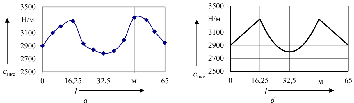
Рисунок 4 – Распределение жесткости контактной подвески в пролете: a – полученное экспериментально; б – принятое для использования в модели
