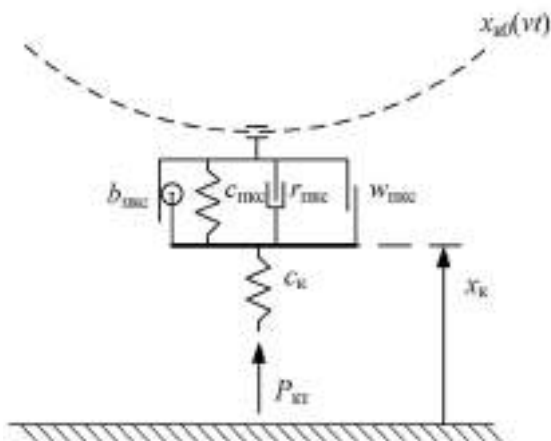
Рисунок 3 – Предлагаемая схема модели контактной подвески
