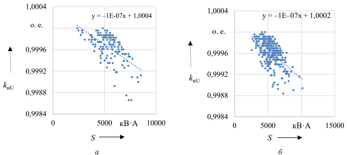
Рисунок 12 – Коэффициент искажения напряжения для шин 0,4 кВ ввода 1 ( a ) и ввода 2 ( б )
