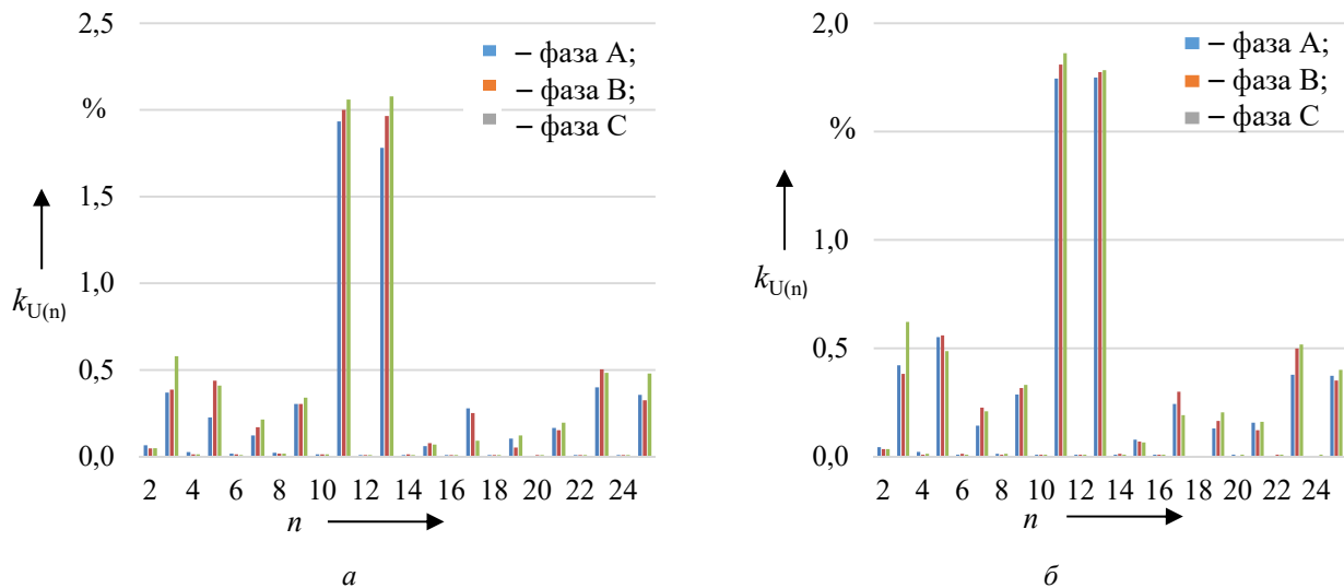
Рисунок 10 – Диаграмма спектра токов по вводу 1-0,4 (а) и по вводу 2-0,4 (б) (значения для фаз А, В и С приведены подряд для каждой из n гармоник)
