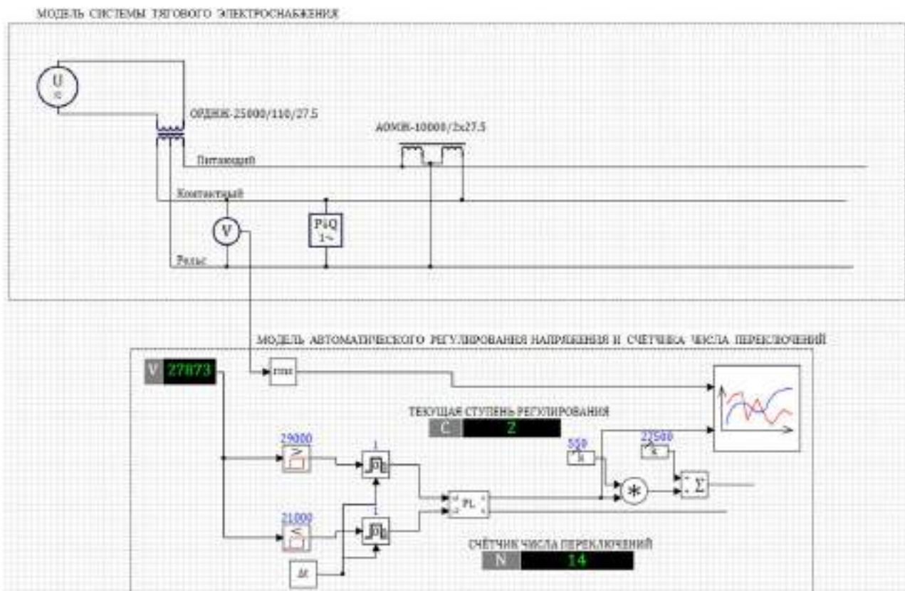
Рисунок 4 – Рабочее окно модели в программном комплексе SimInTech
