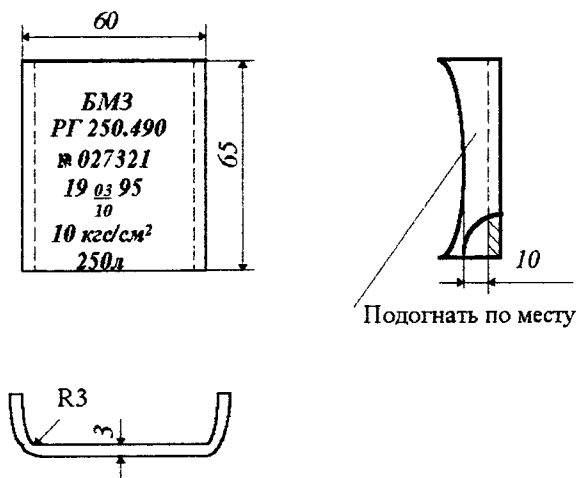
Рисунок 3 - Образец таблички с указанием паспортных данных резервуара
