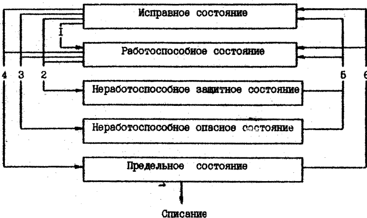
Рис.3. Схема основных состояний и событий: 1 — повреждение; 2 — защитный отказ; 3 — опасный отказ; 4 — переход системы в предельное состояние из-за неустранимого нарушения требований безопасности, снижения эффективности эксплуатации, морального старения и других факторов; 5 — восстановление; 6 — ремонт
