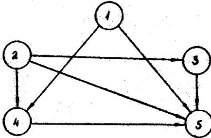
Рис.8. Граф безопасных ложных переходов электрической централизации
