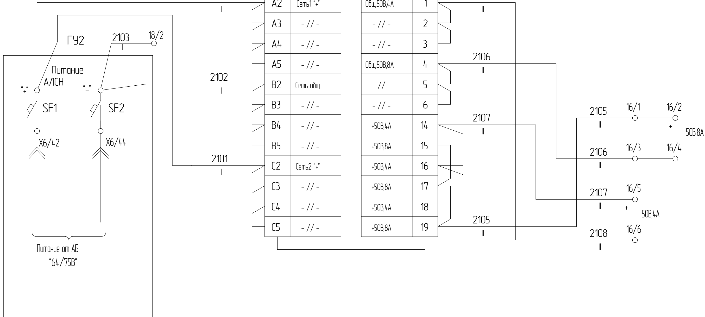
Электрическая схема теплобоза
