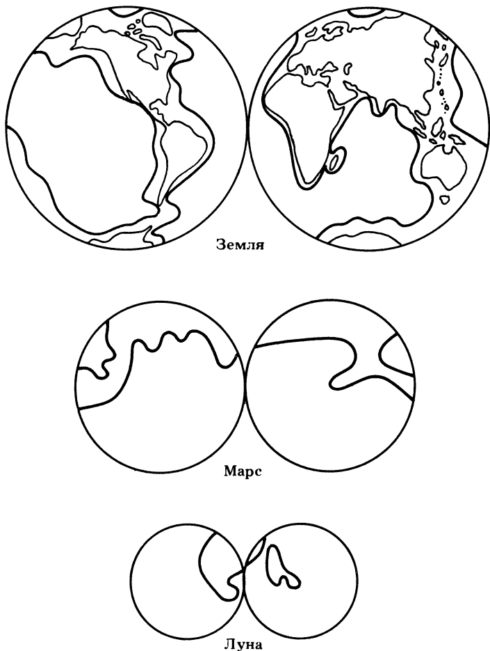
Рис. 3. Тектоническая асимметрия Земли, Марса и Луны.
