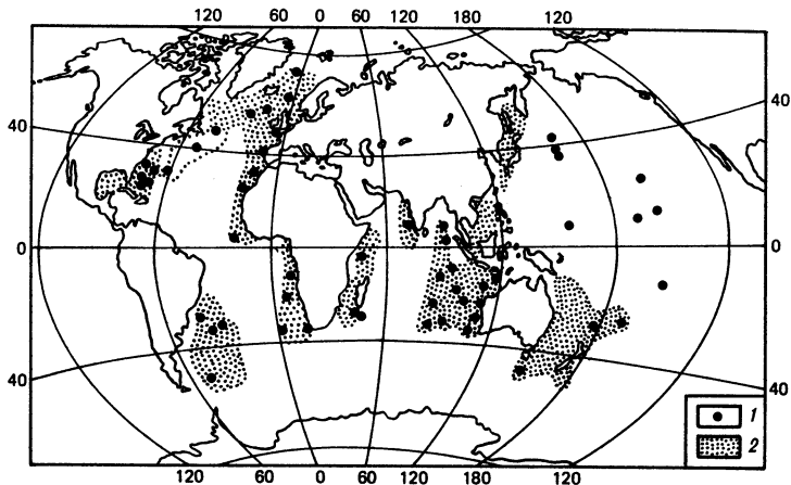
Рис. 1. Крупное (1—5 км) опускание океанического дна в верхнемеловую эпоху и в кайнозое.
