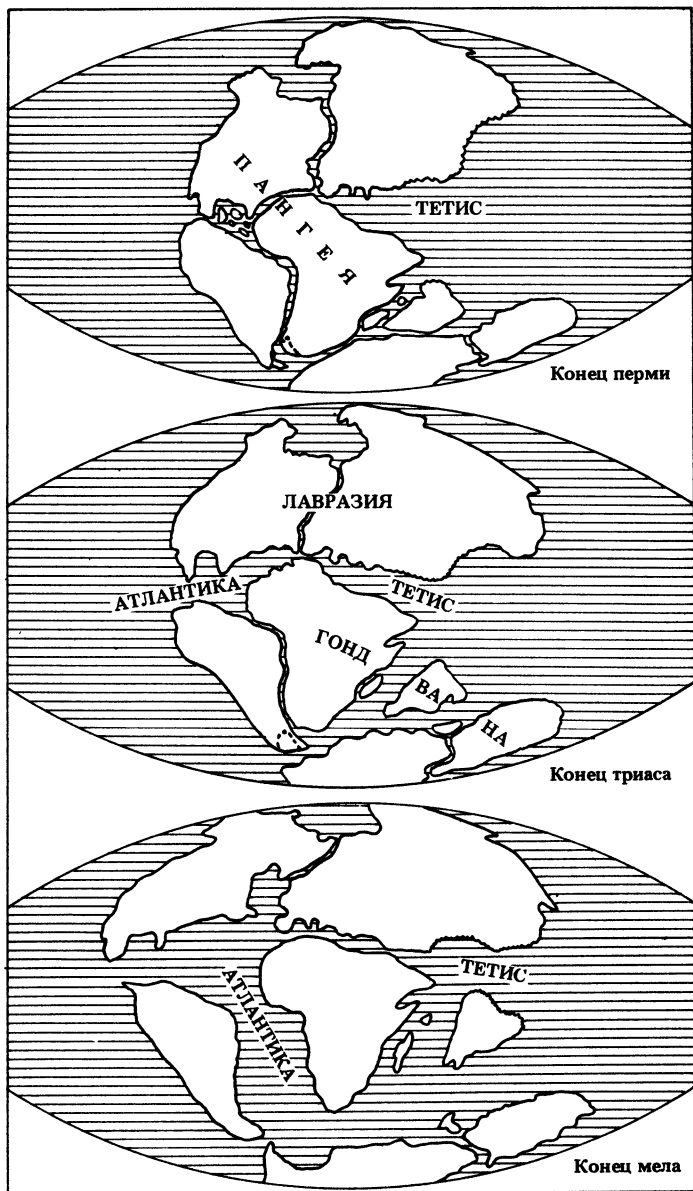
Рис. 10. Реконструкция распада Пангеи и Гондваны.
