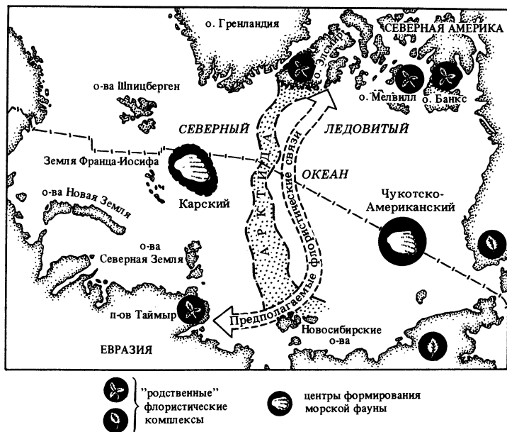
Рис. 15. Схематическое изображение вероятностных флористических связей в период существования Арктиды и современное положение фаунистических комплексов (по Я. Я. Гакkelю и Л. С. Говорухе).
