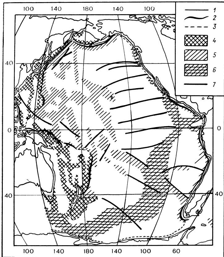
Рис. 4. Схема крупнейших форм рельефа дна Тихого океана (по Г. Б. Удинцеву).
