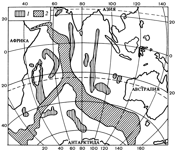
Рис. 8. Геоморфология дна Индийского океана.
