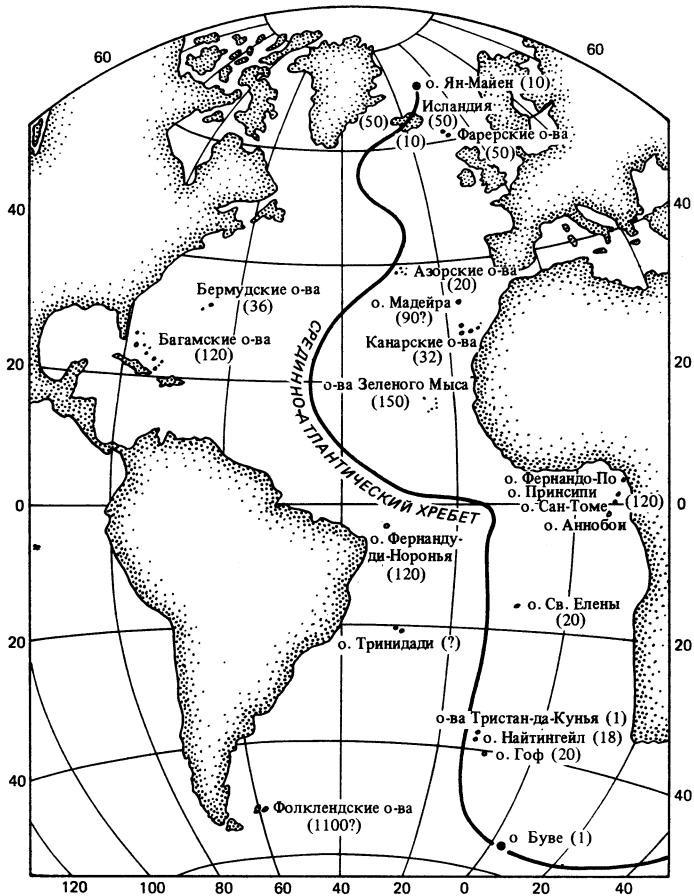
Рис. 13. Возраст островов Атлантики (в миллионах лет).
