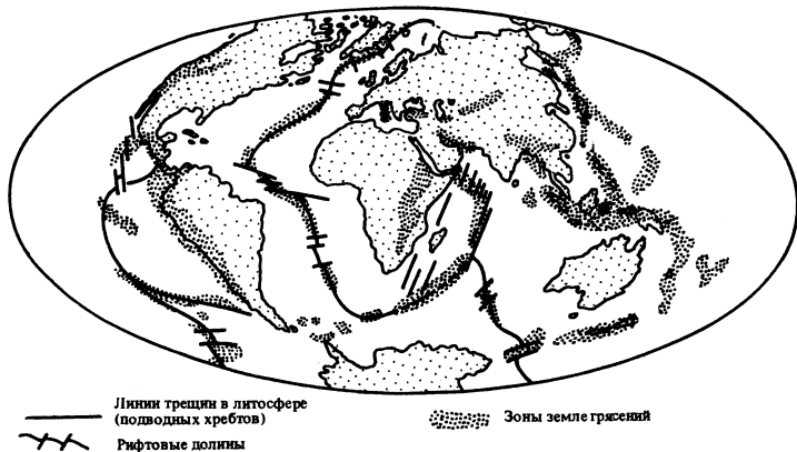
Рис. 11. Глобальная система срединных океанических хребтов.
