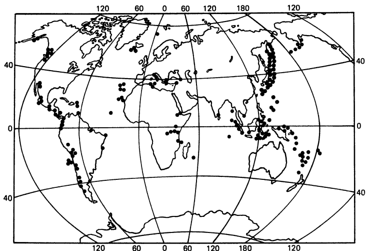
Рис. 5. Расположение действующих вулканов на земном шаре.
