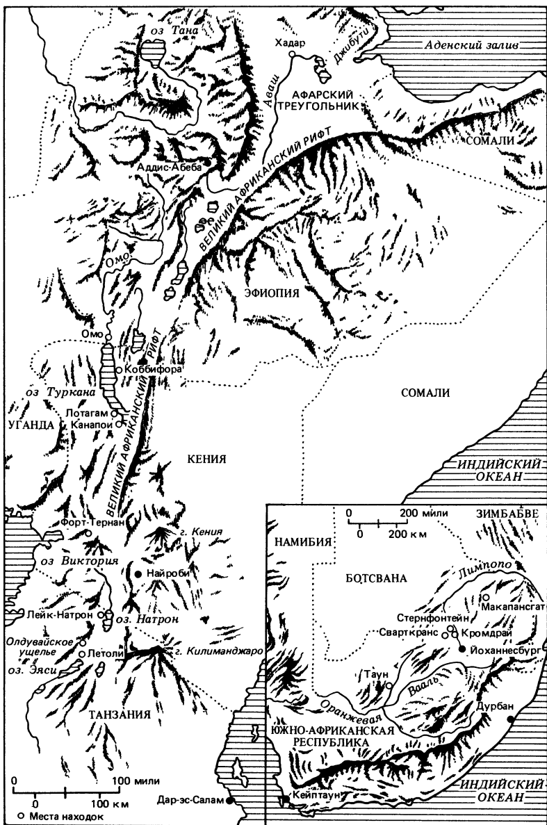
Рис. 7. Великий Восточно-Африканский рифт и места находок предков человека в Восточной и Южной Африке.
