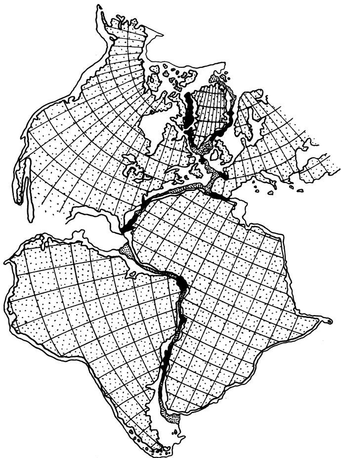
Рис. 9. Сходство очертаний континентов планеты.
