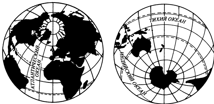
Рис. 2. «Материковое» и «океаническое» полушария Земли.
