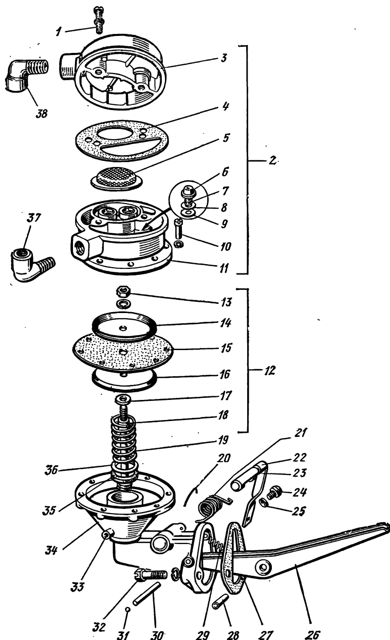
Рис. 15. Бензиновый насос
