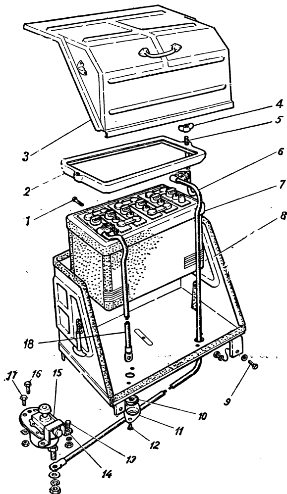
Рис. 52. Аккумуляторная батарея
