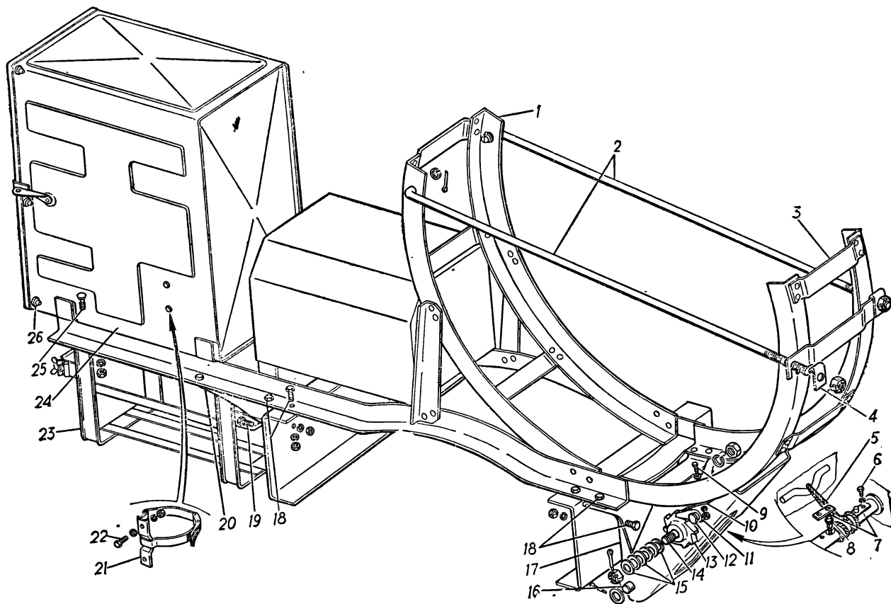
Рис. 41. Держатель запасного колеса
