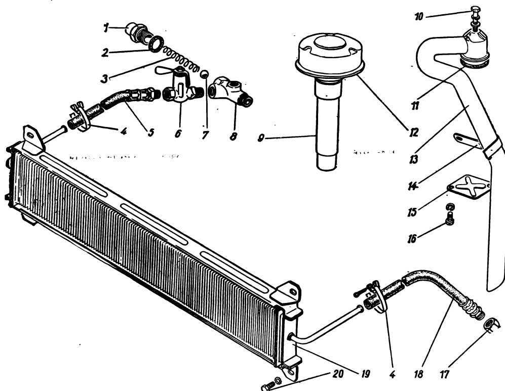
Рис. 9. Масляный радиатор и вентиляция картера Примечание. Поз. 9 см. в подгруппе 1009
