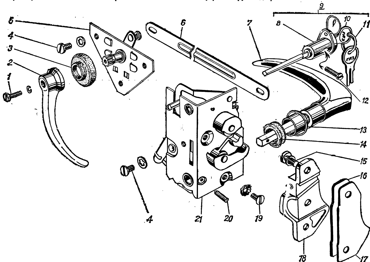
Рис. 79. Замок и ручки двери
