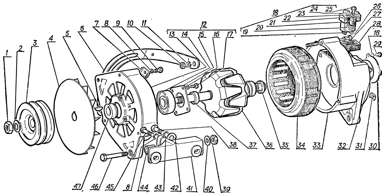
Рис. 51. Генератор
