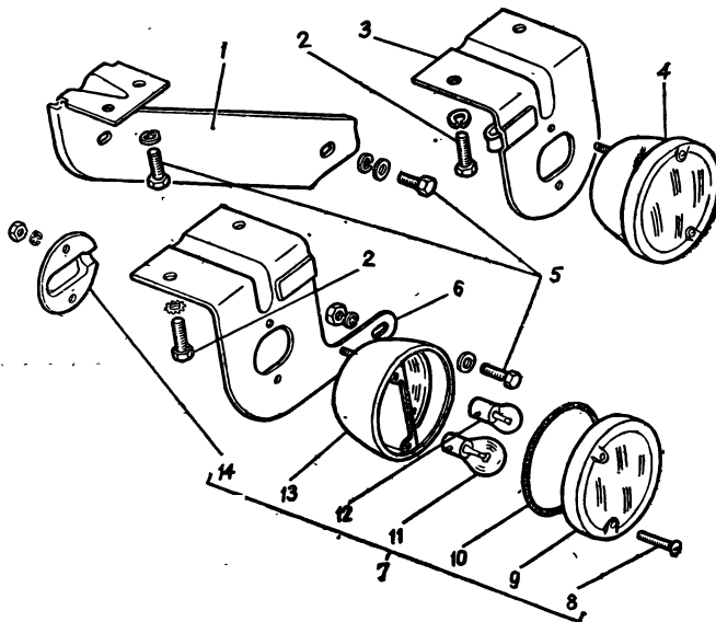
Рис. 59. Задний фонарь
