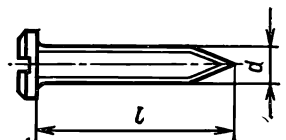
Винты с плоской головкой самонарезающие для металла и пластмассы
