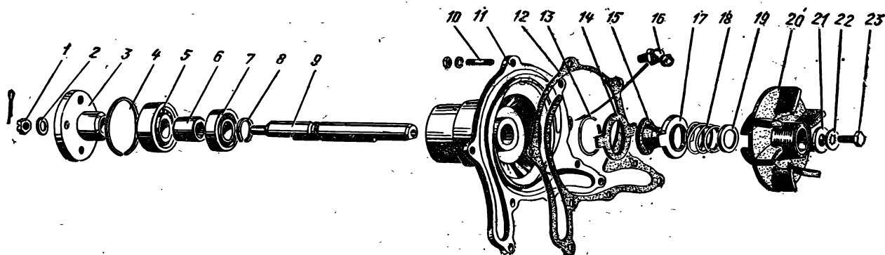
Рис. 23. Водяной насос
