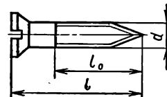
Шуруп по дереву с потайной головкой
