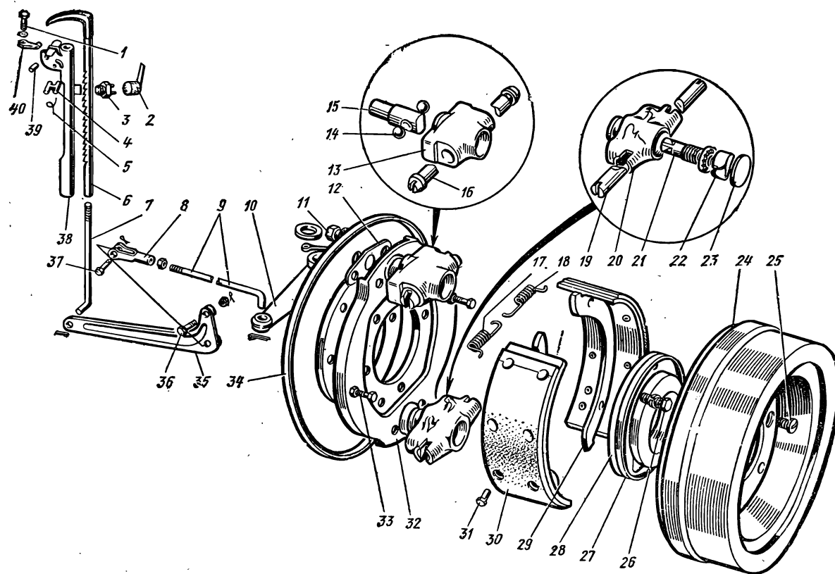
Рис. 48. Стояночный тормоз и управление
