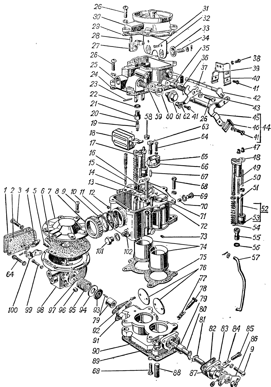
Рис. 16. Карбюратор
