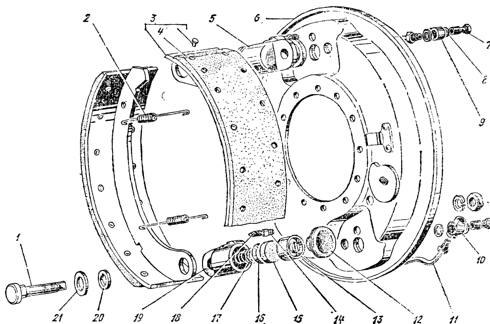
Рис. 44. Передние рабочие тормоза
