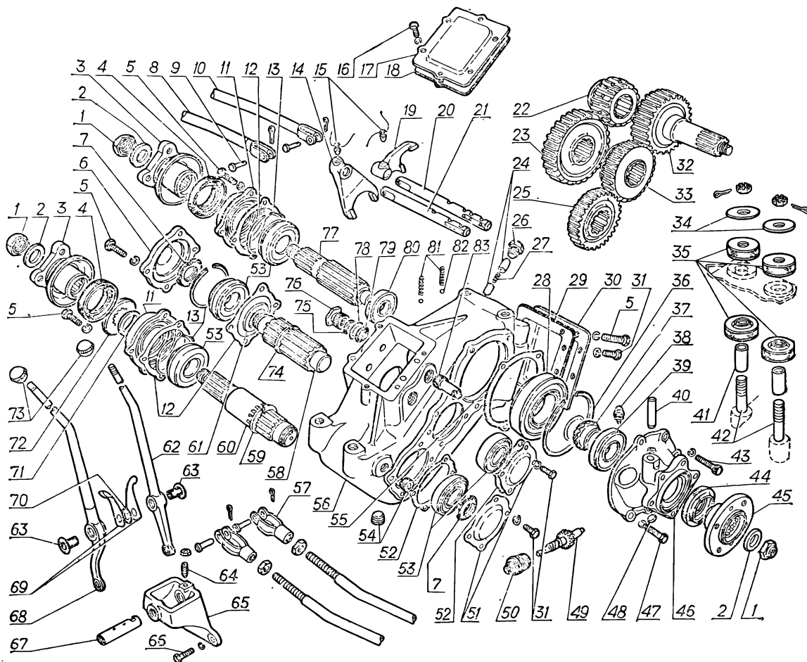
Рис. 29. Раздаточная коробка
