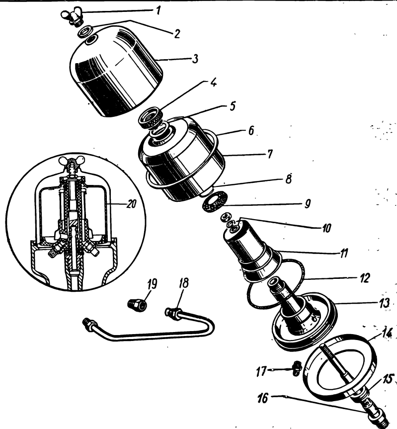
Рис. 11. Фильтр центробежной очистки масла
