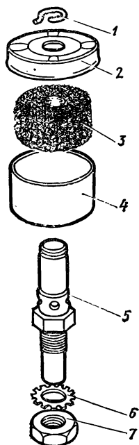
Рис. 50. Воздушный фильтр гидровакуумного усилителя тормозов
