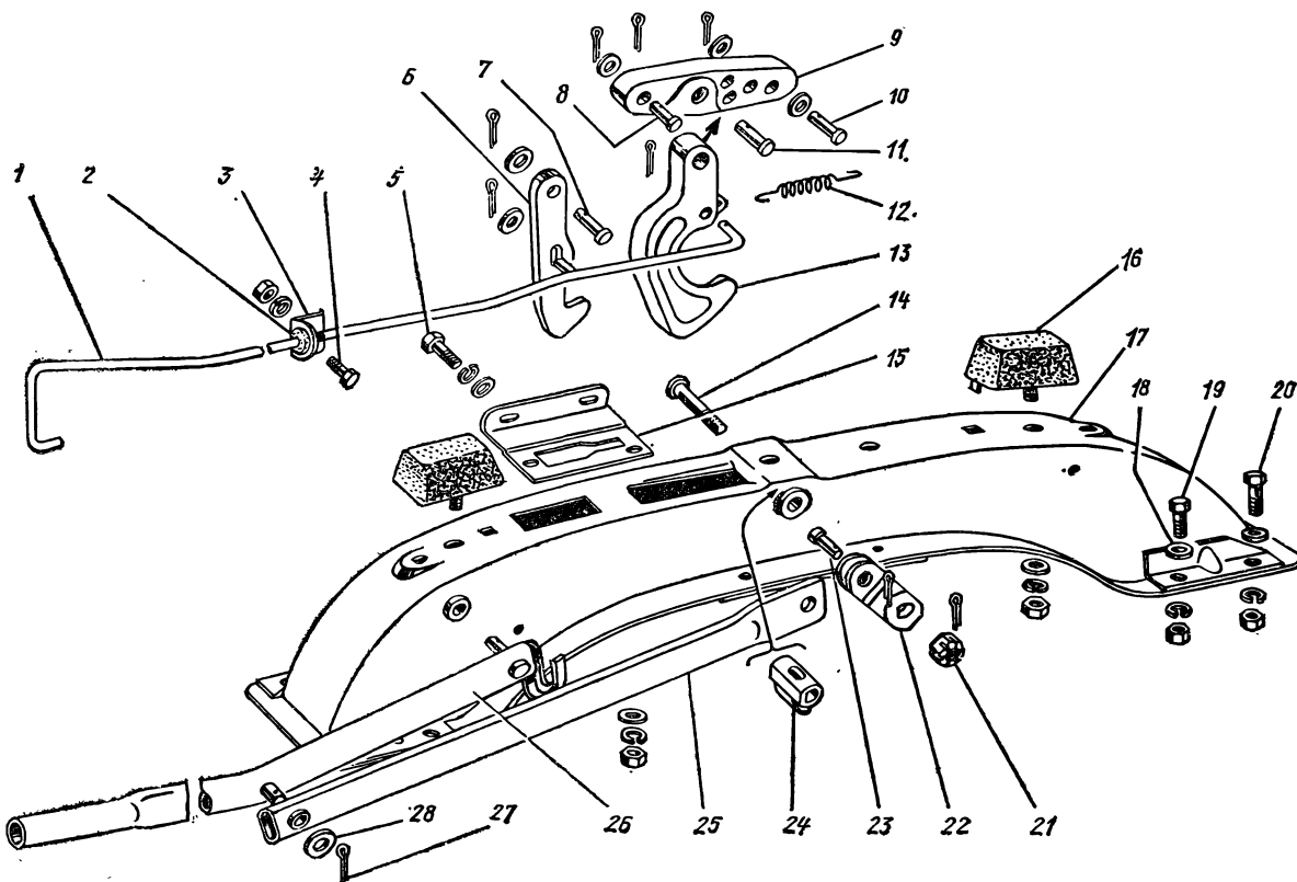
Рис. 73. Крепление кабины
