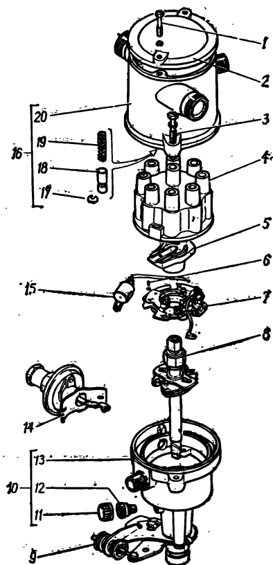
Рис. 56. Распределитель автомобиля ГАЗ-66-05
