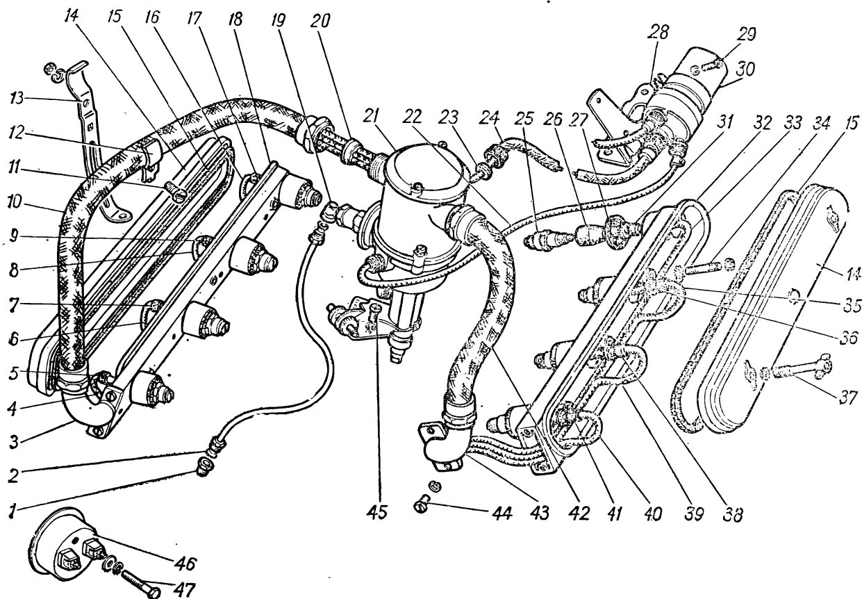
Рис. 55. Катодка зажигания, распределитель, свечи и провода зажигания автомобиля ГАЗ-66-05
