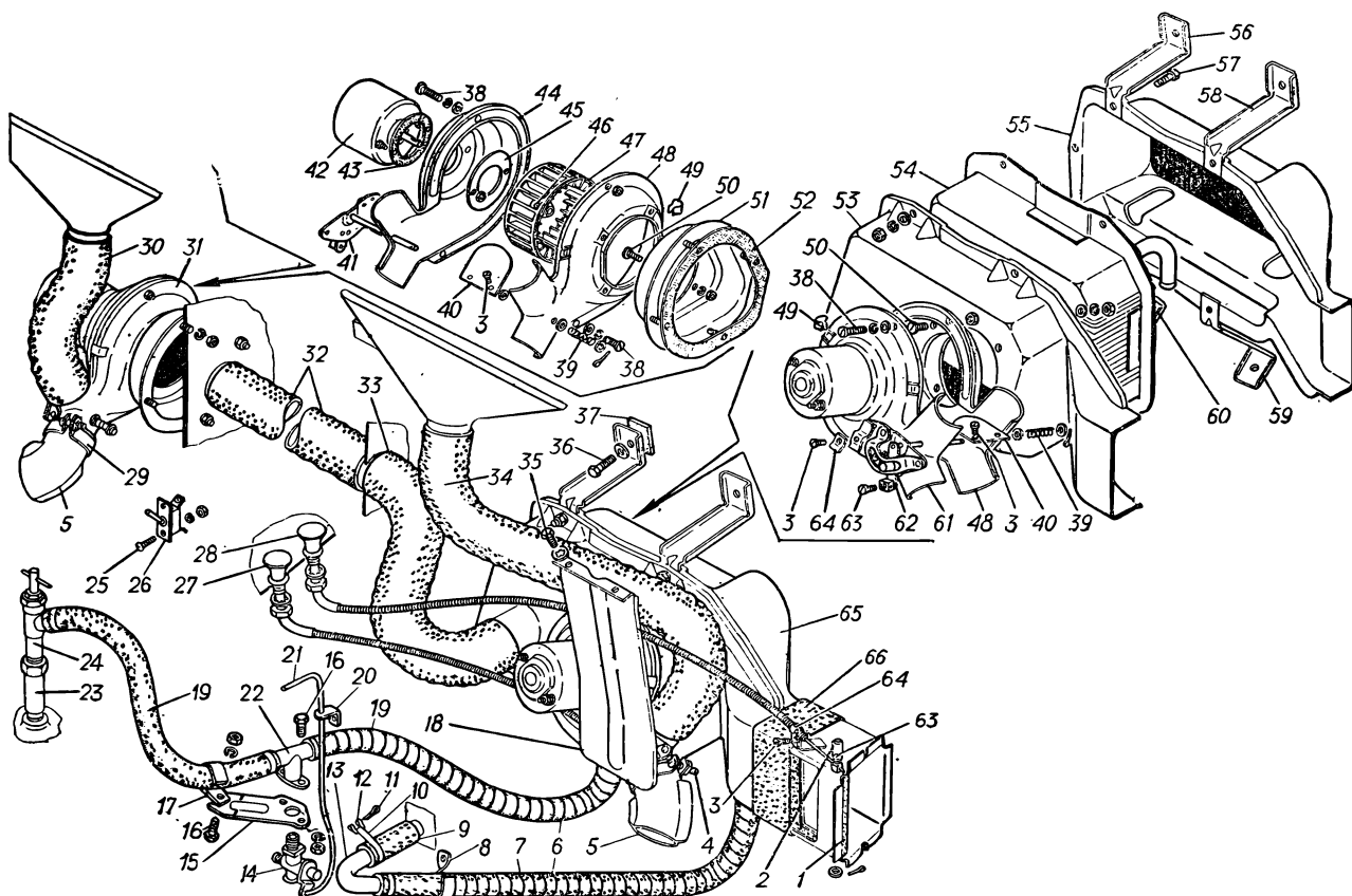
Рис. 81. Вентиляция и отопление
