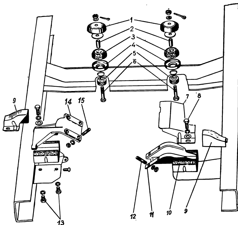
Рис. 2. Подвеска двигателя
