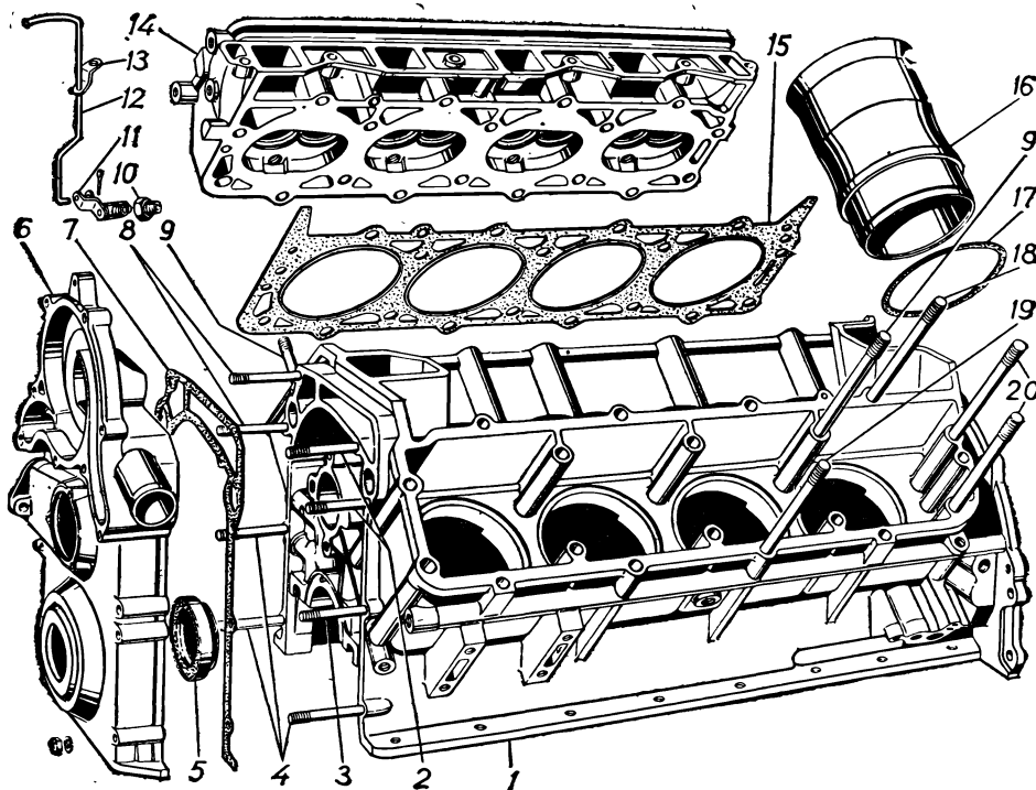
Рис. 3. Блок и головка блока цилиндров
