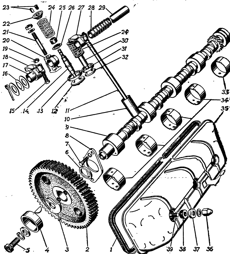
Рис. 5. Распределительный вал, клапаны и толкатели
