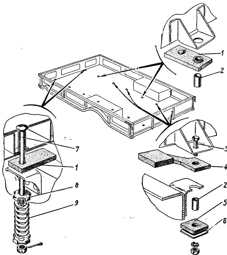
Рис. 85. Крепление платформы
