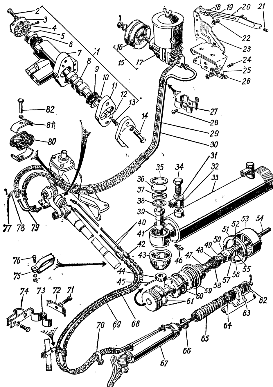
Рис. 43. Гидроусилитель руля
