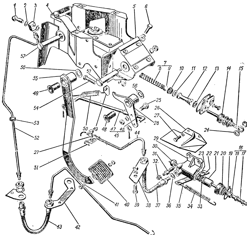
Рис. 26. Привод выключения сцепления
