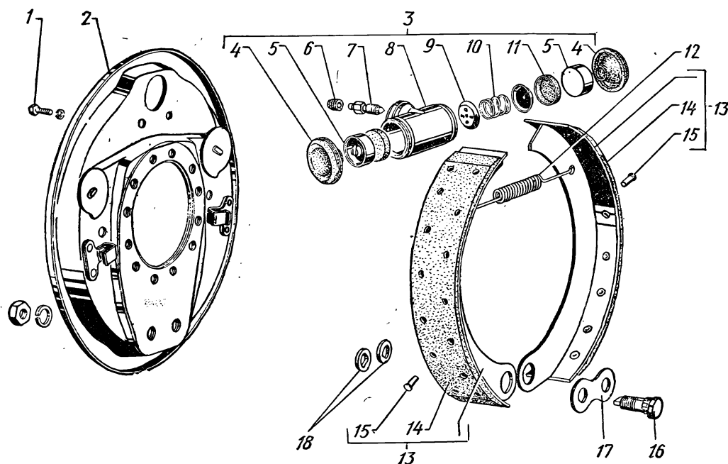
Рис. 45. Задние рабочие тормоза
