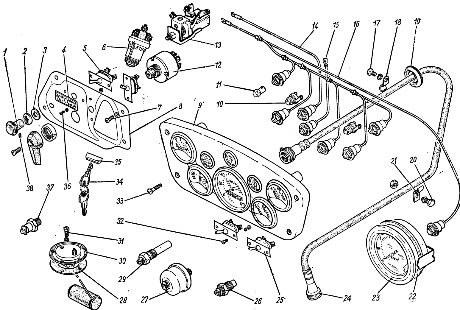
Рис. 62. Щиток приборов
