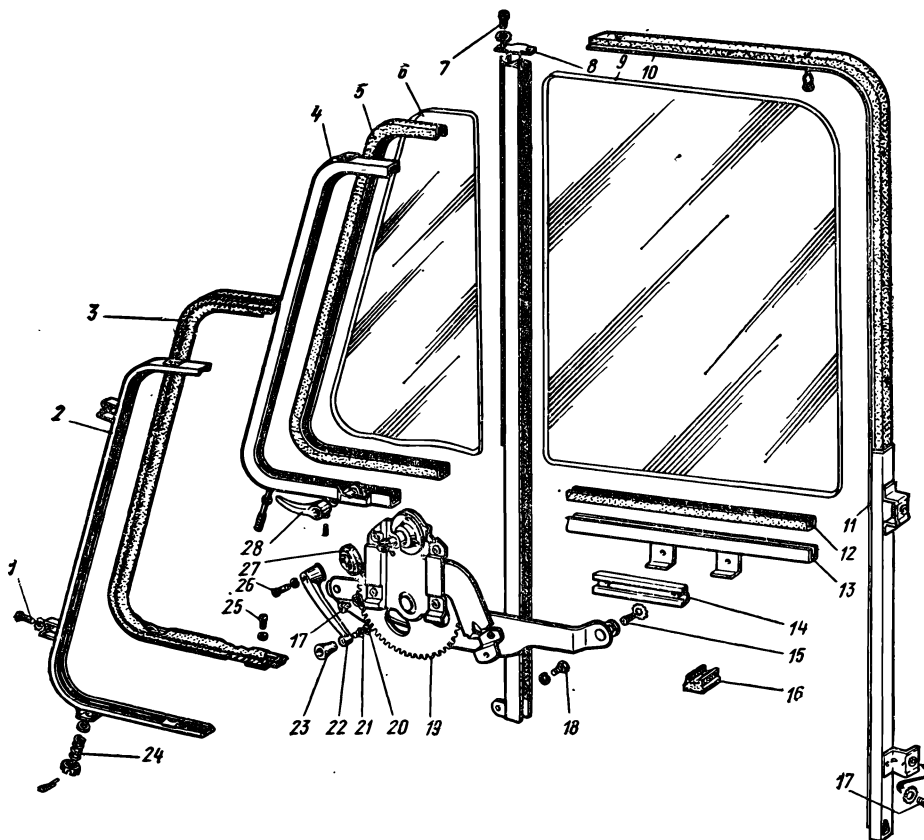
Рис. 78. Окно двери и стеклоподъемник
