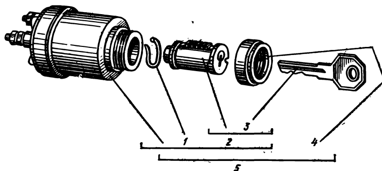
Рис. 53. Выключатель зажигания
