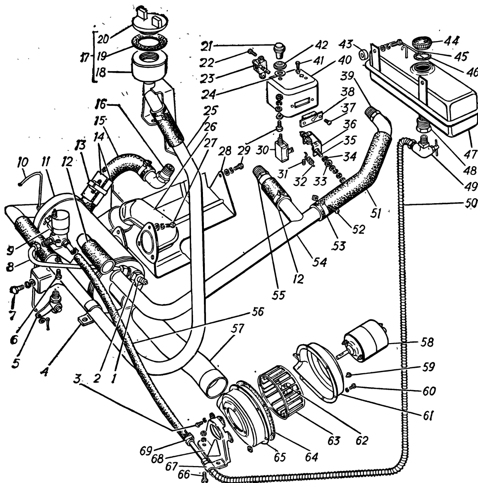
Рис. 10. Пусковой подогреватель
