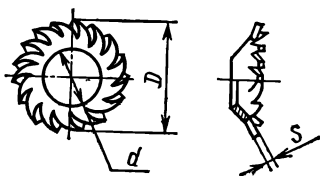
Шайба пружинная коническая с наружными зубьями
