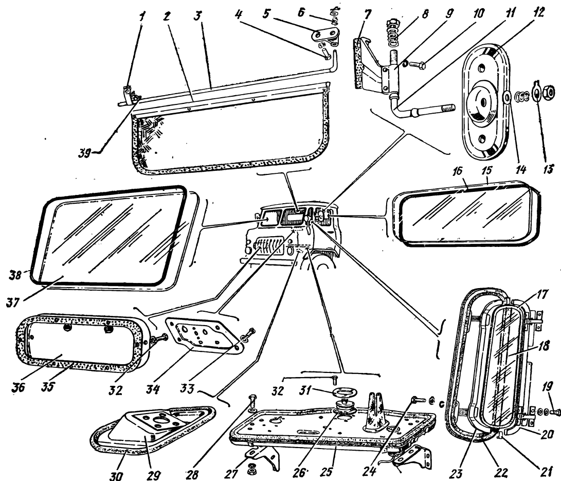
Рис. 74. Детали пола, передка и принадлежности кабины
