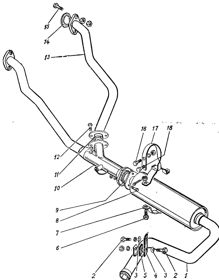
Рис. 21. Глушитель
