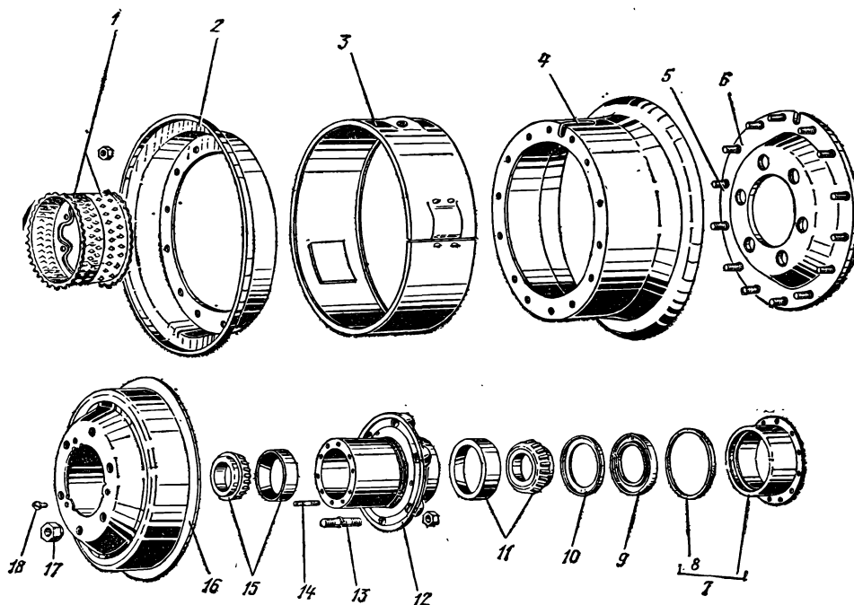
Рис. 40. Колеса и ступицы
