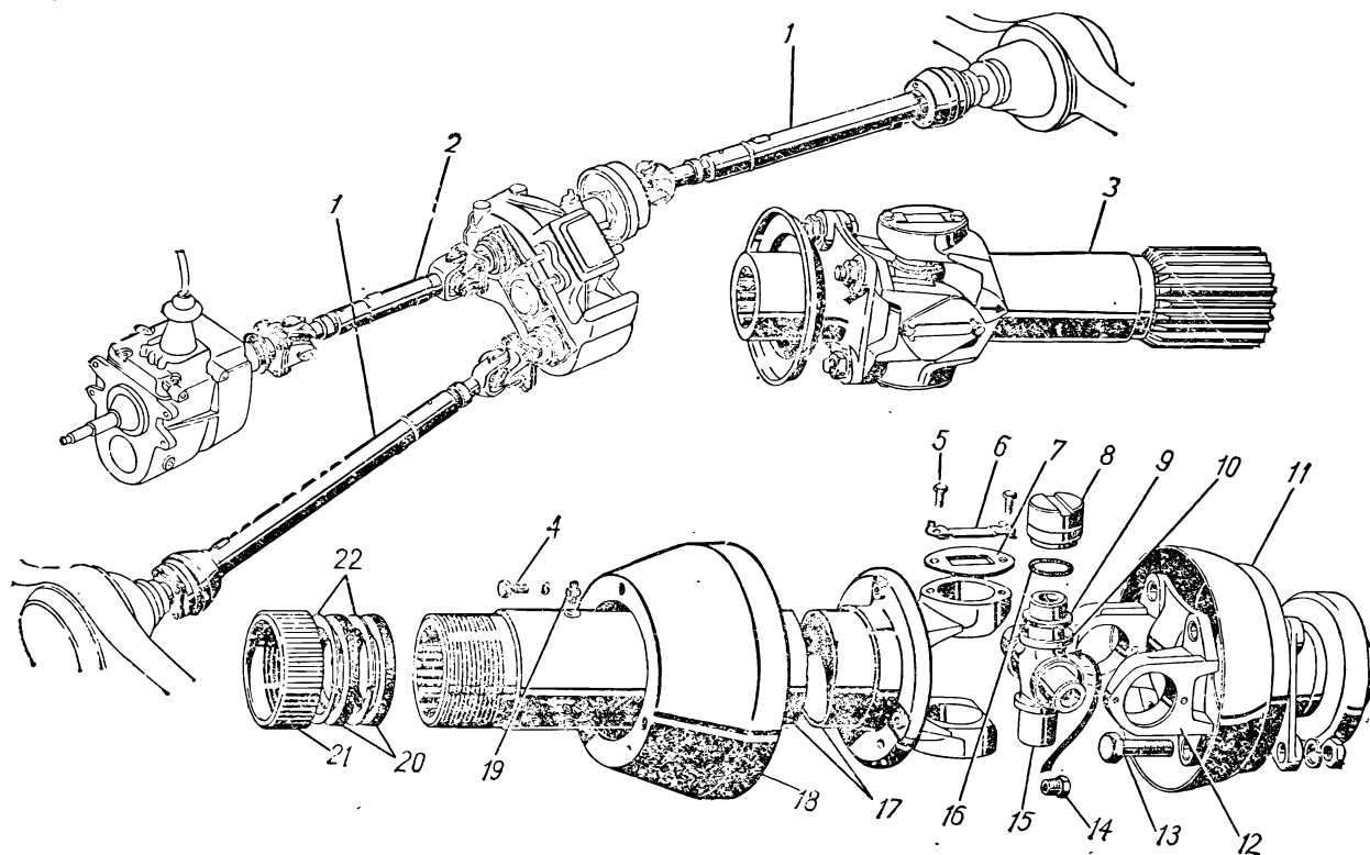
Рис. 30. Карданные валы
