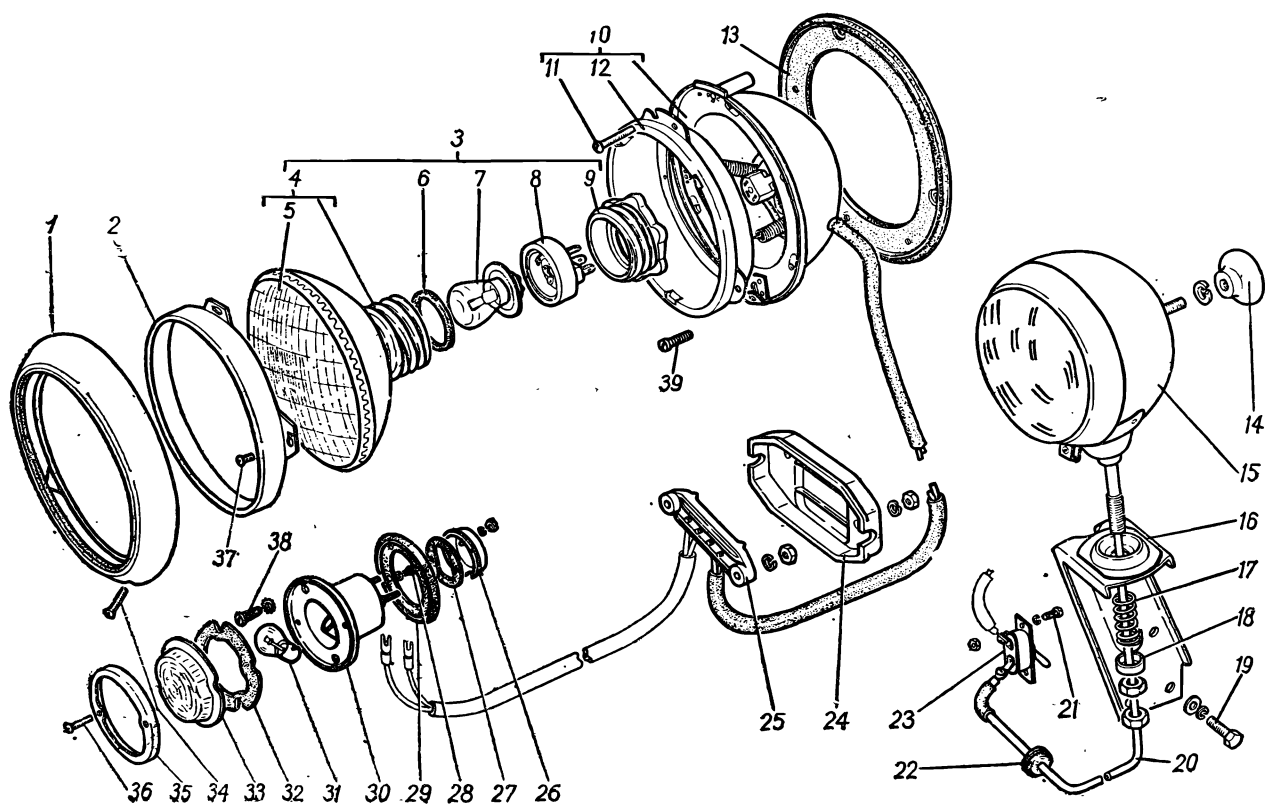
Рис. 58. Фары и подфарники
