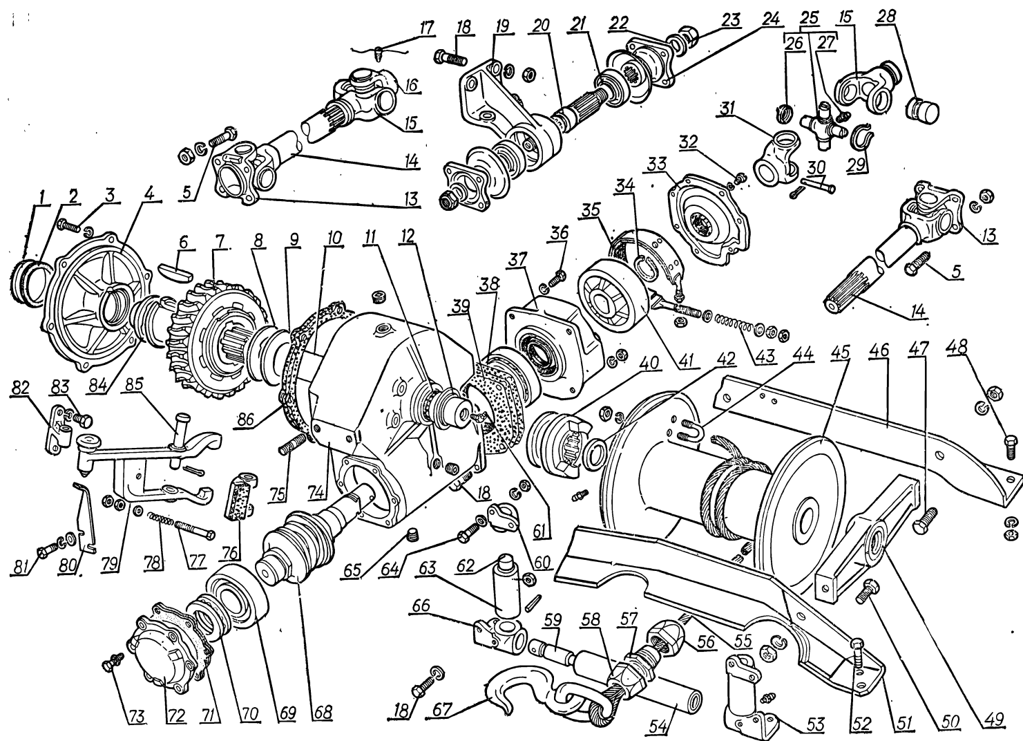
Рис. 70. Лебедка
