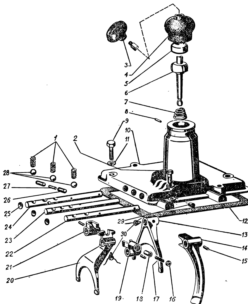
Рис. 28. Механизм переключения передач
