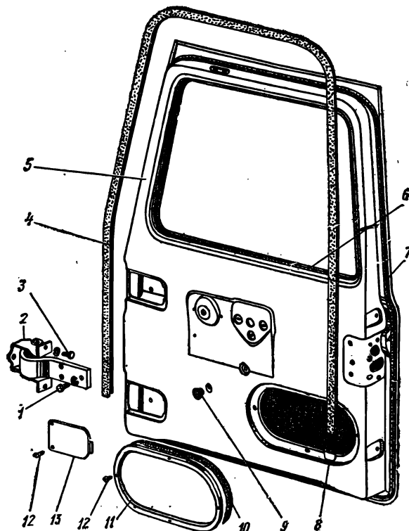
Рис. 77. Дверь
