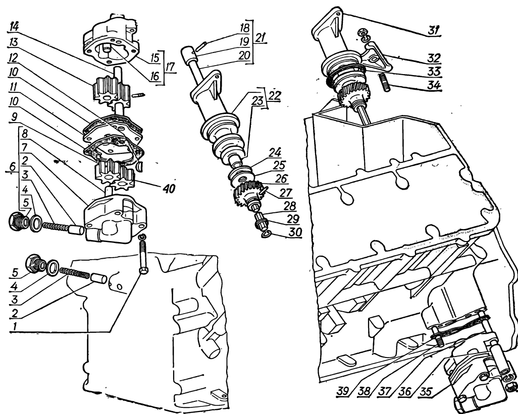
Рис. 8. Масляный насос и привод распределителя
