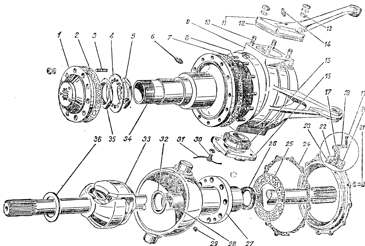
Рис. 33. Поворотные кулаки
