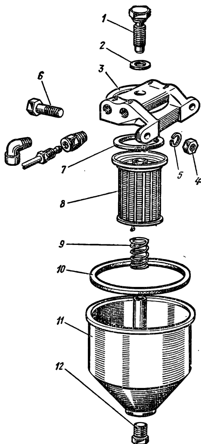
Рис. 14. Бензиновый отстойник
