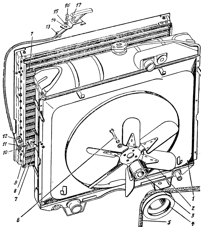
Рис. 24. Вентилятор и жалюзи радиатора
