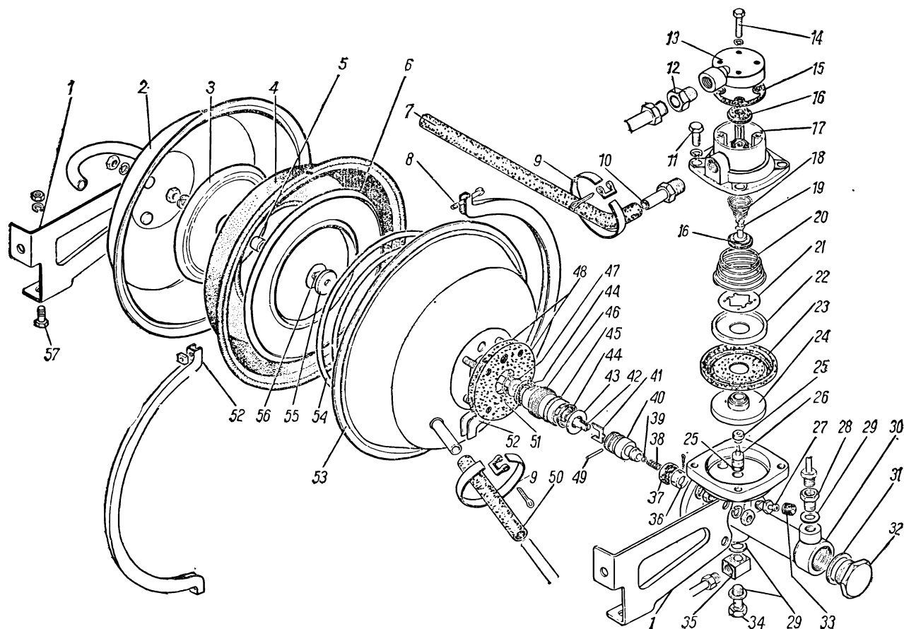
Рис. 49. Гидровакуумный усилитель тормозов и клапан управления
