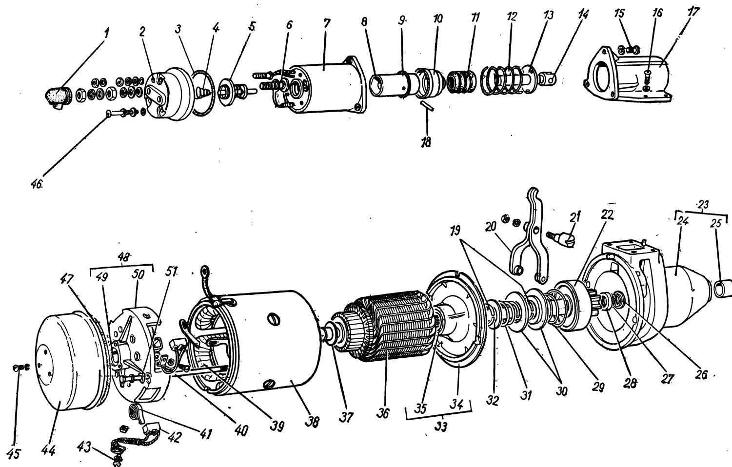
Рис. 57. Стартер
