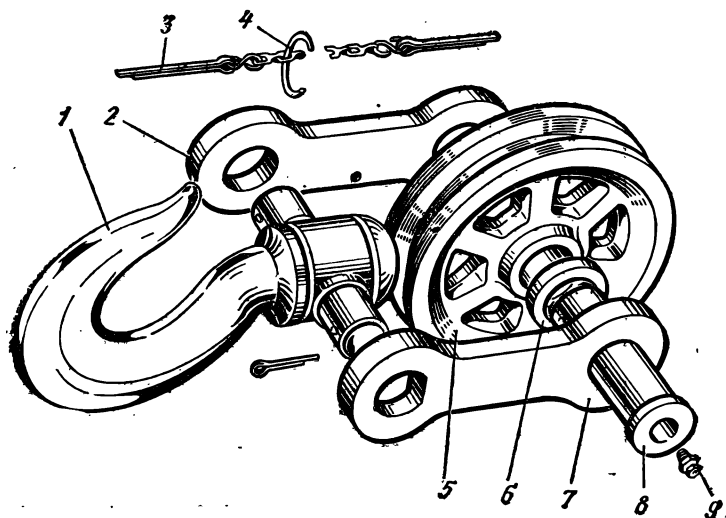
Рис. 71. Блок лебедки
