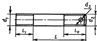
Шпилька с отверстием в стержне
