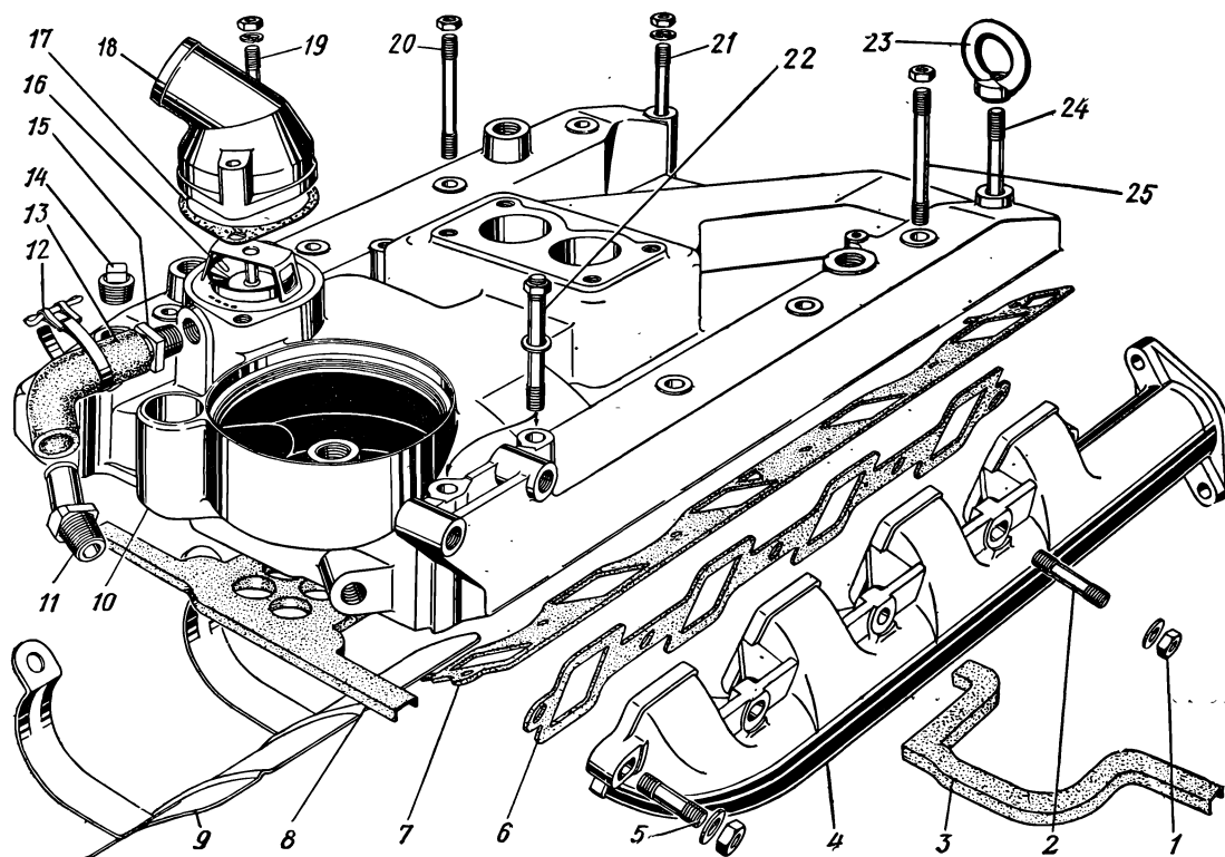
Рис. 6. Газопровод
