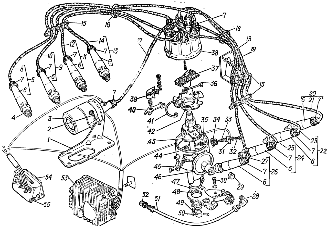
Рис. 54. Катушка зажигания, распределитель, свечи и провода зажигания автомобиля ГАЗ-66-01
