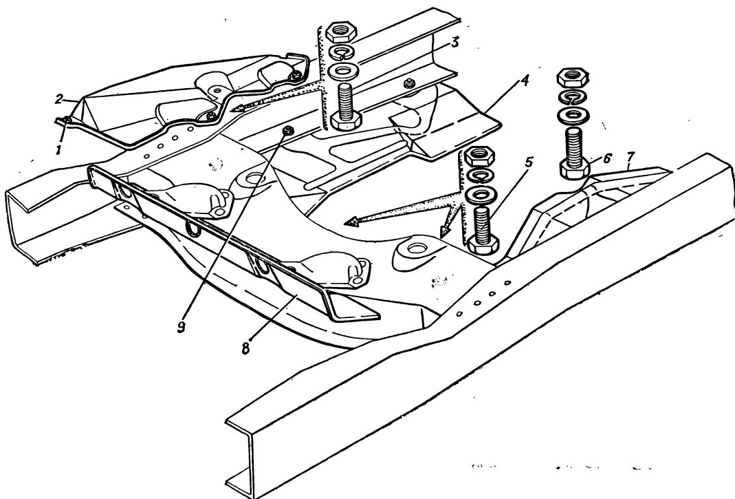
Рис. 35. Брызговики
