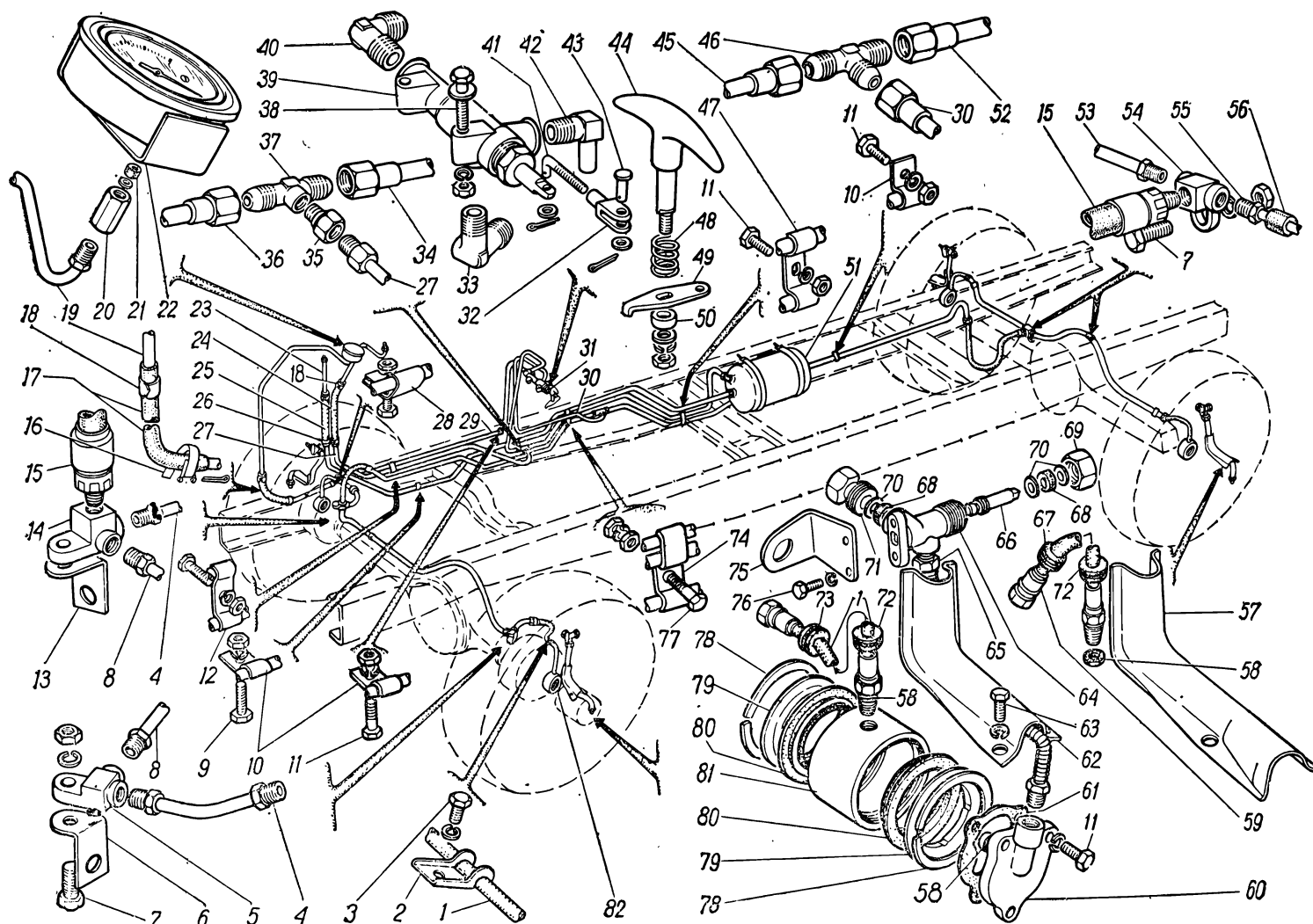
Рис. 68. Кран управления давлением системы подкачки шин, подвод воздуха к шинам и трубопроводы
