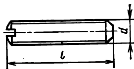
Винт установочный с коническим концом
