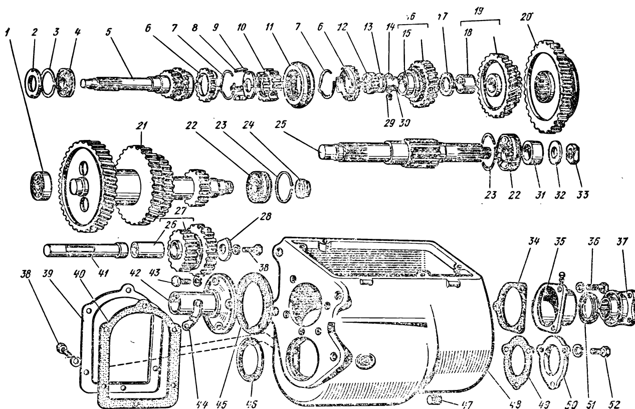
Рис. 27. Коробка передач
