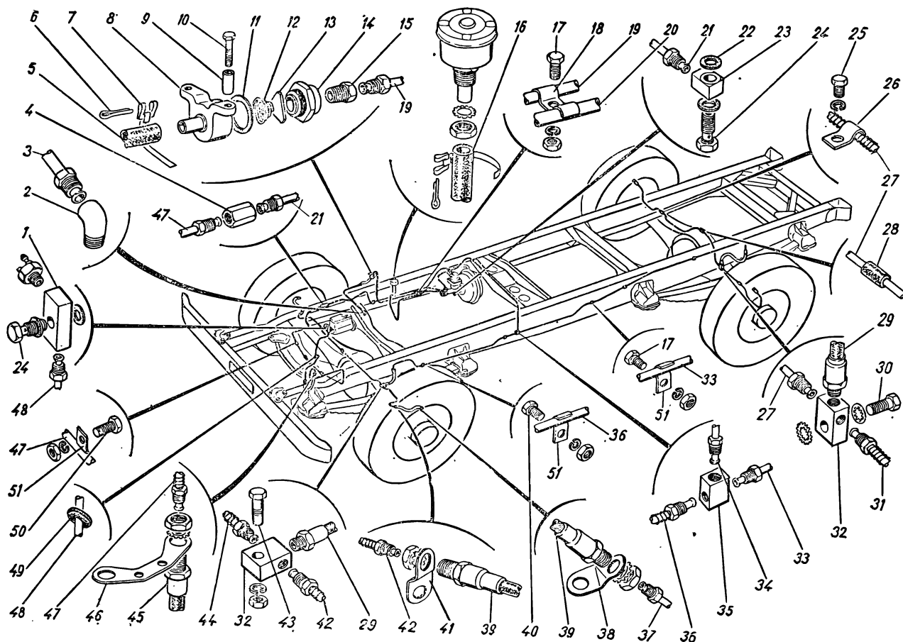
Рис. 47. Трубопроводы гидротормозов
