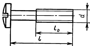
Винты с плоской головкой
