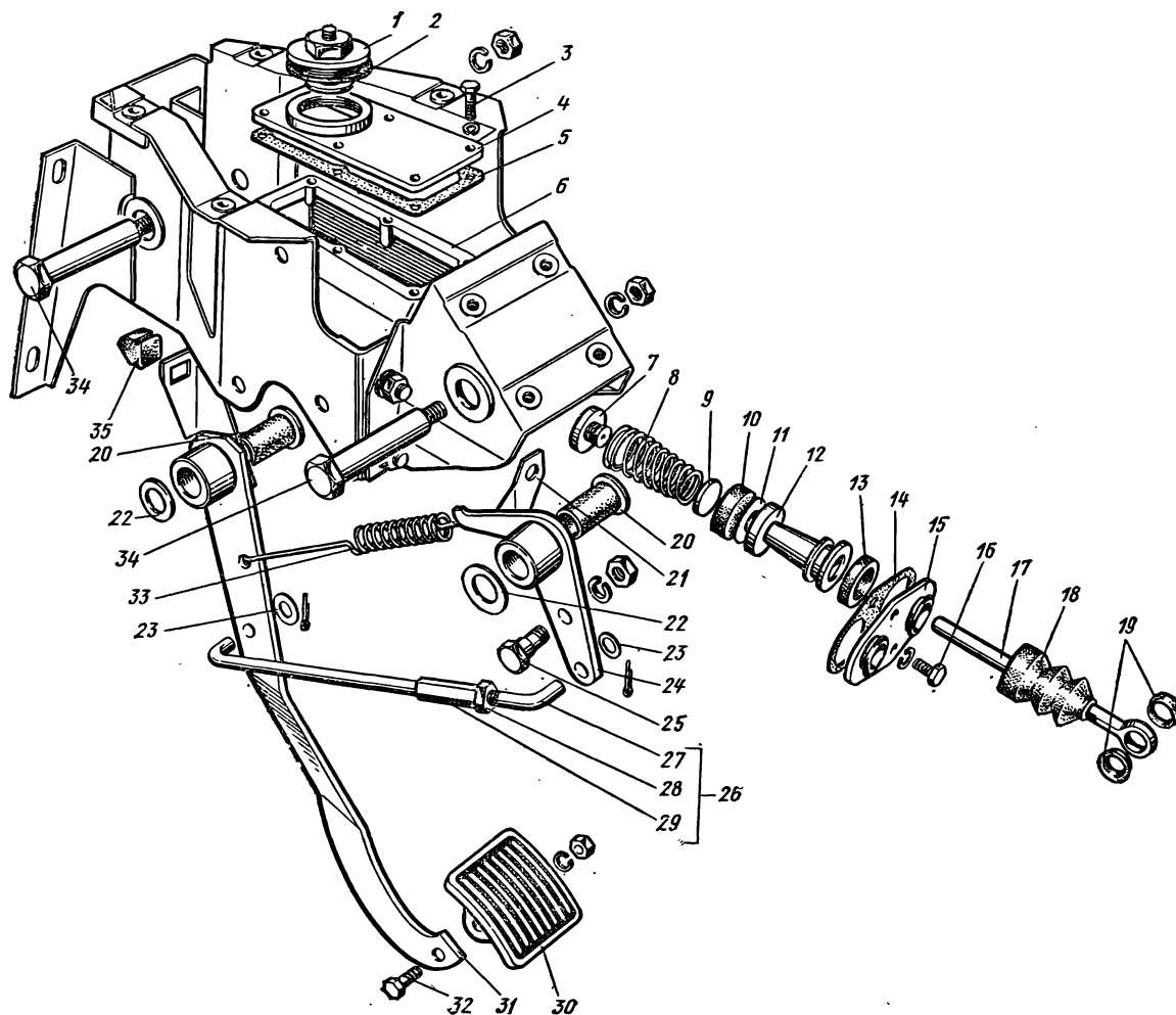
Рис. 46. Главный цилиндр тормоза, педаль и привод
