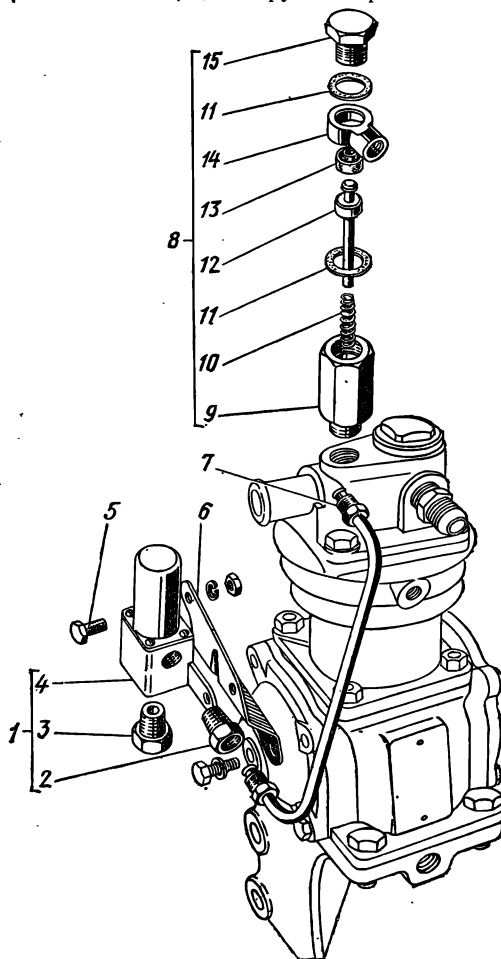
Рис. 69. Разгрузочный цилиндр компрессора и регулятор давления
