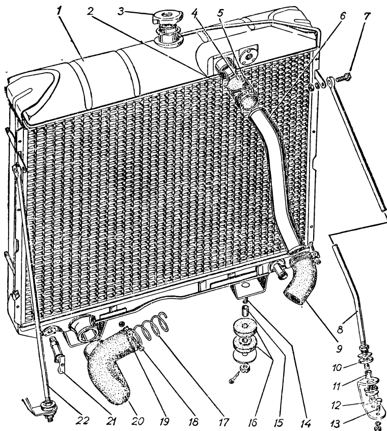
Рис. 22. Радиатор
