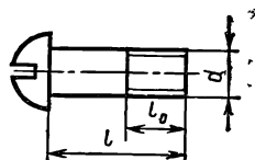
Винты с полукруглой головкой
