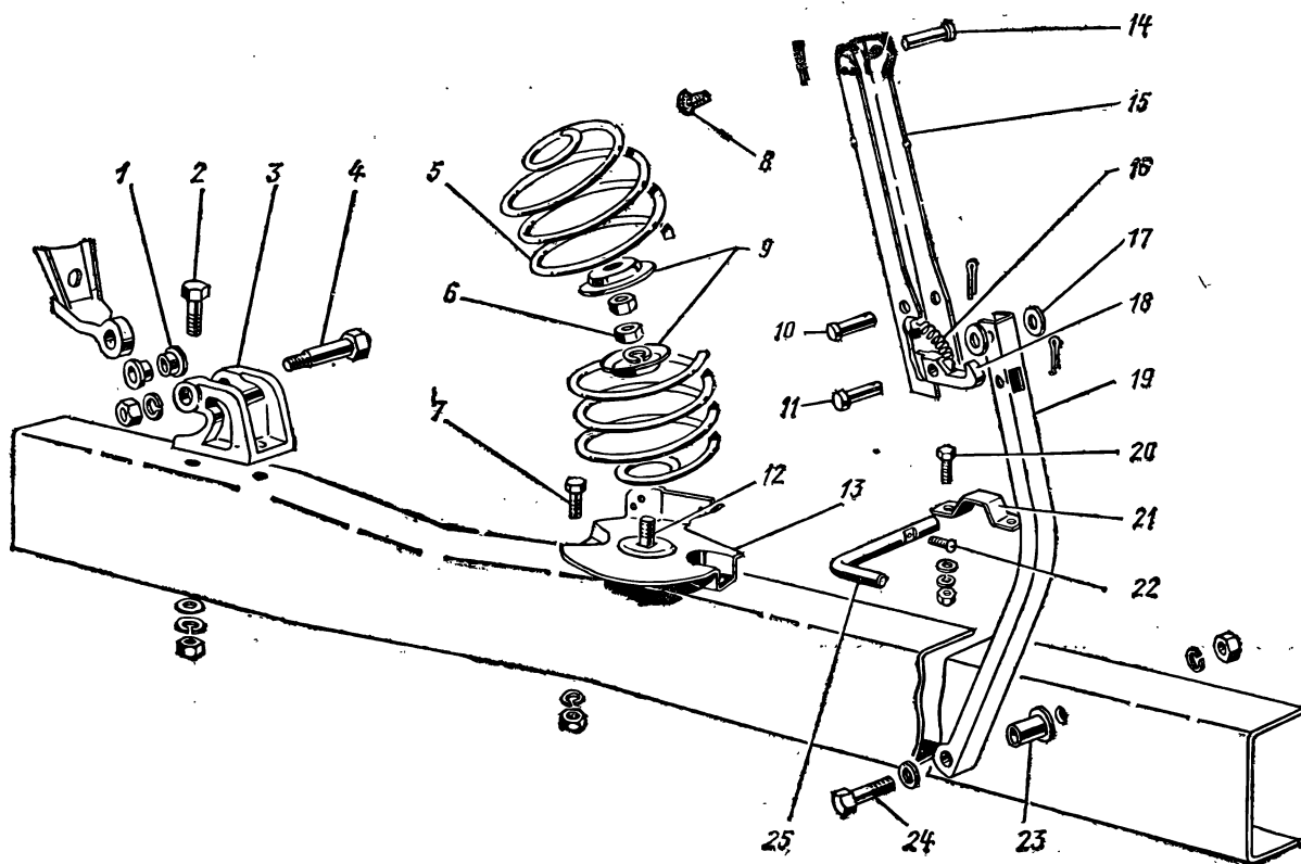
Рис. 72. Механизм опрокидывания кабины Примечание. Поз. 20 см. в подгруппе 5101
