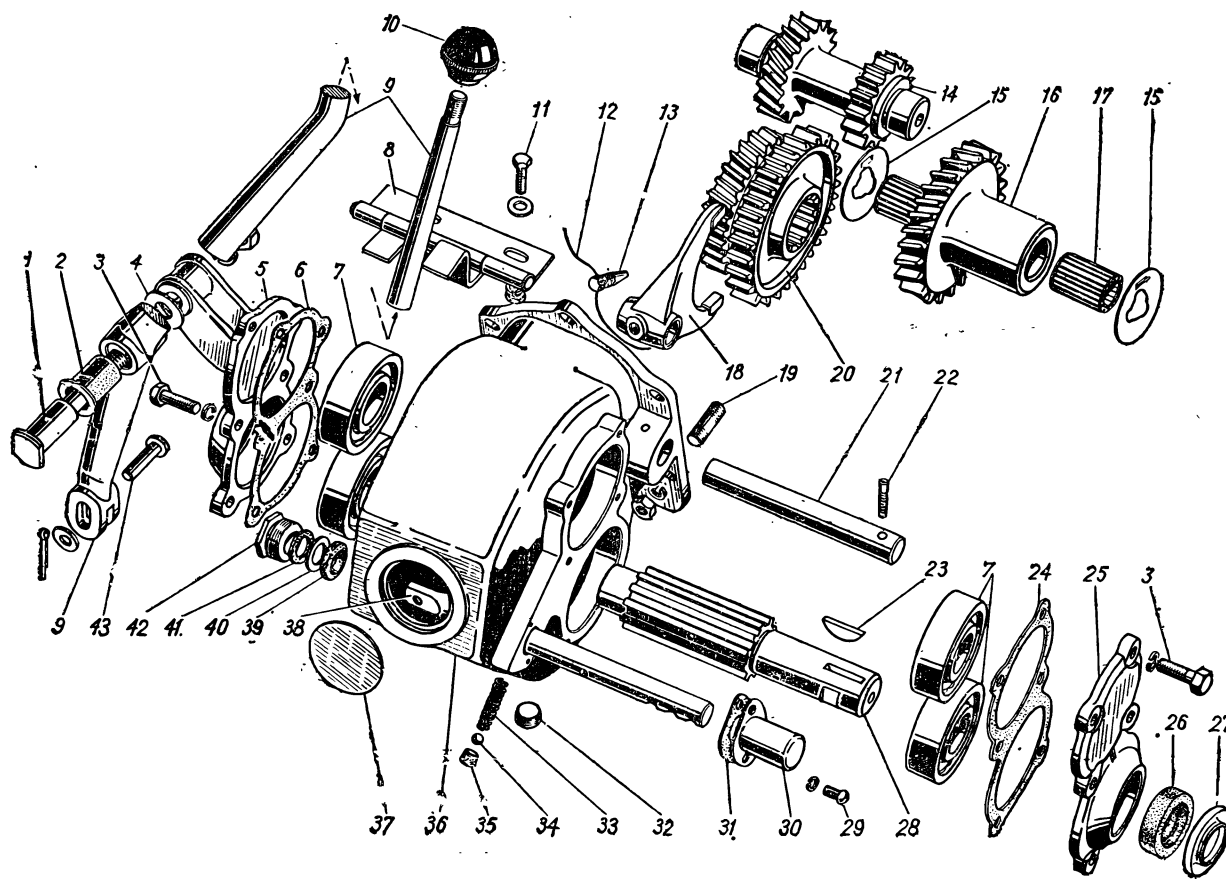
Рис. 66. Коробка отбора мощности
