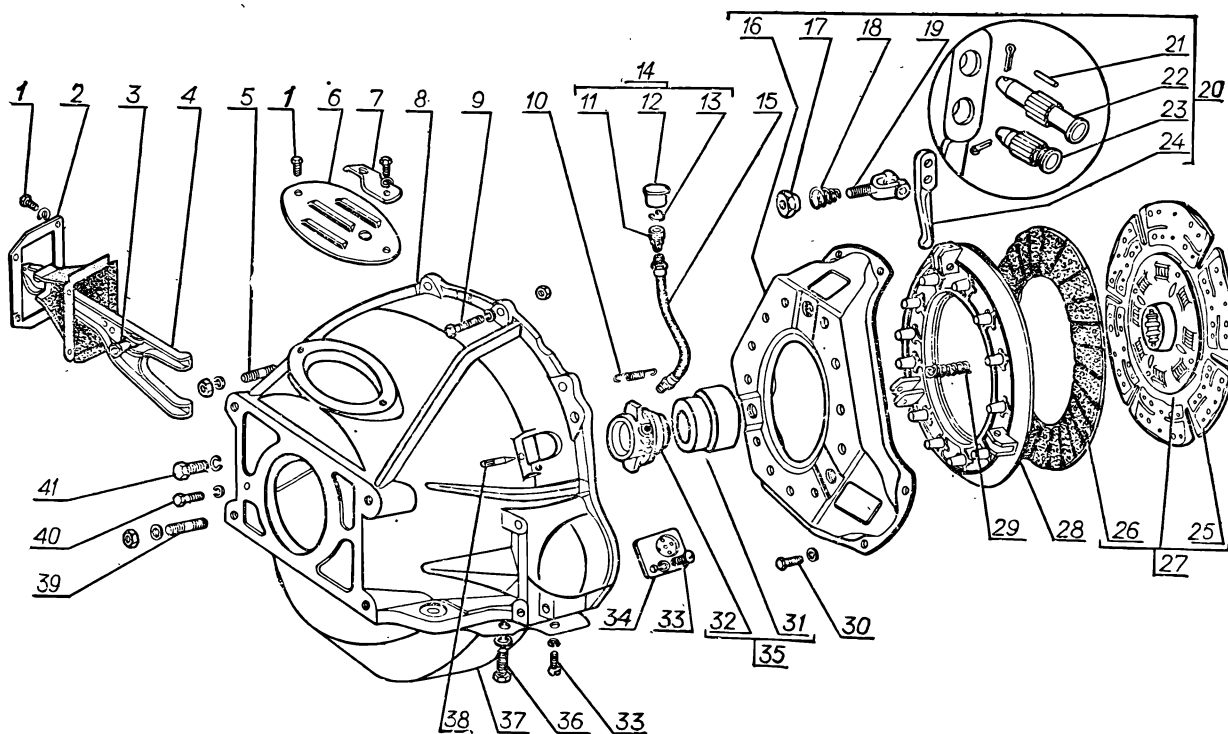
Рис. 25. Сцепление
