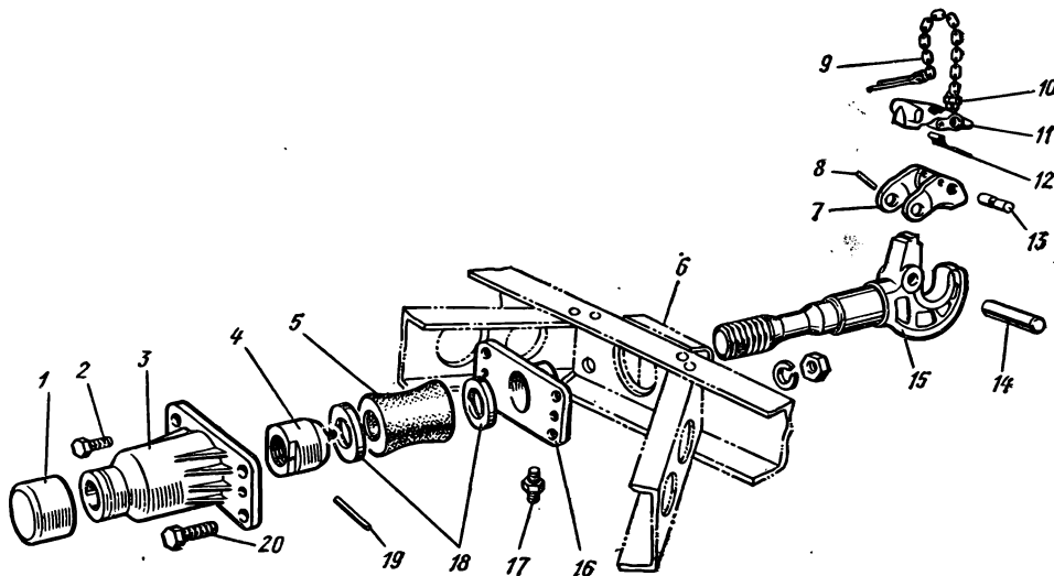
Рис. 36. Буксирный прибор
