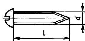
Винт с полукруглой головкой самонарезающий для металла и пластмассы
