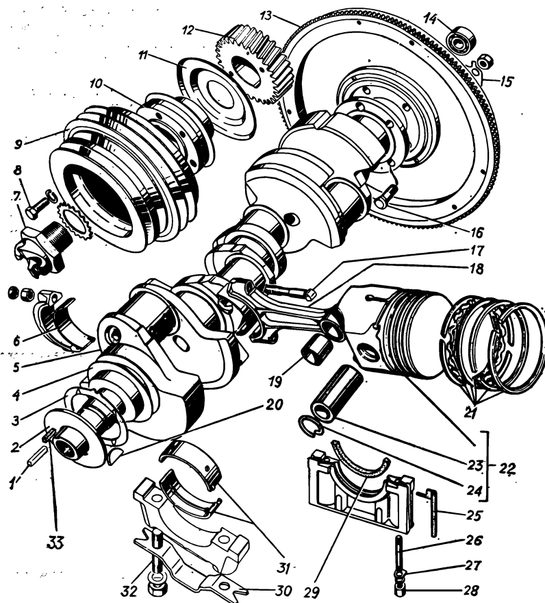
Рис. 4. Коленчатый вал, поршни и шатуны
