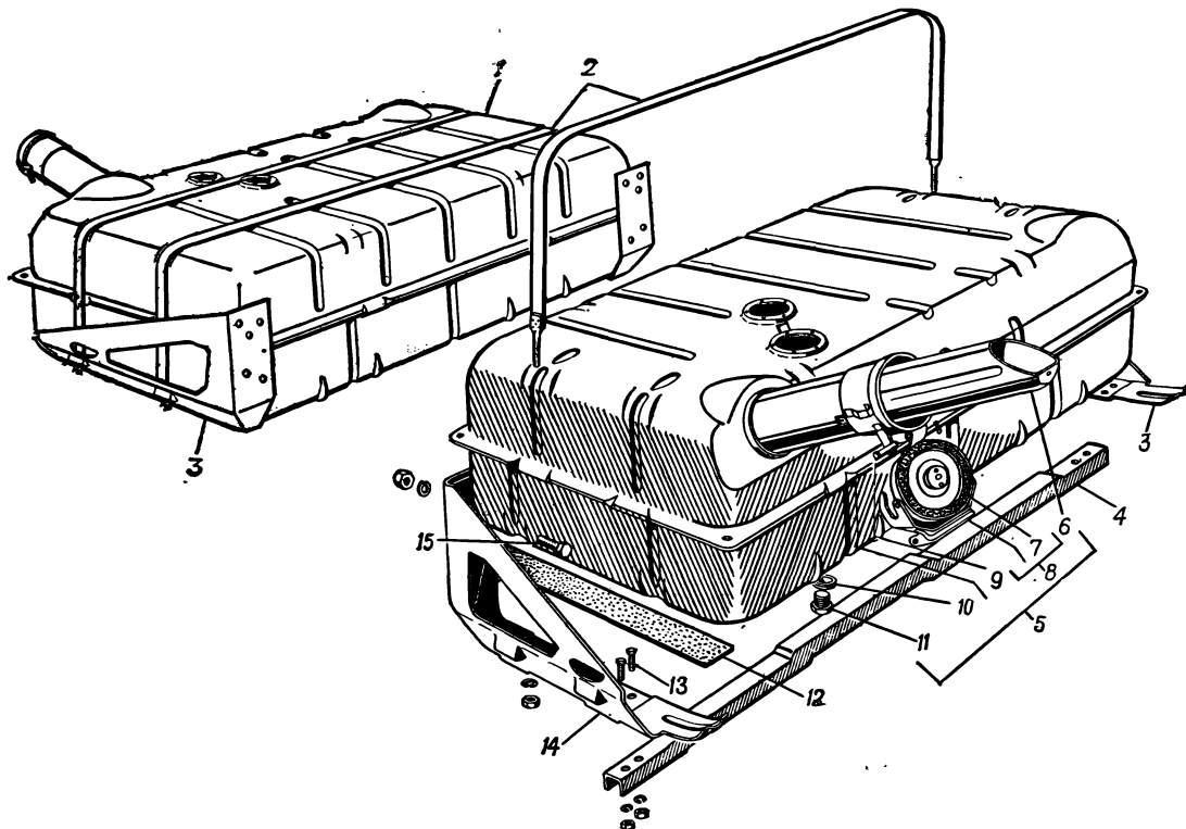
Рис. 12. Бензиновый бак
