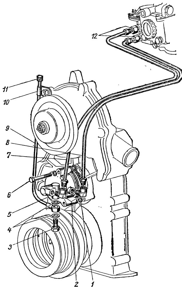
Рис. 19. Пневмоцентробежный ограничитель оборотов
