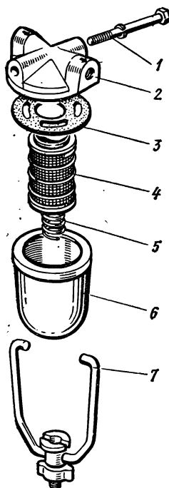
Рис. 20. Фильтр тонкой очистки топлива
