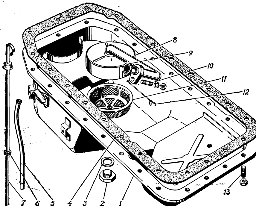
Рис. 7. Масляный картер и маслоприемник
