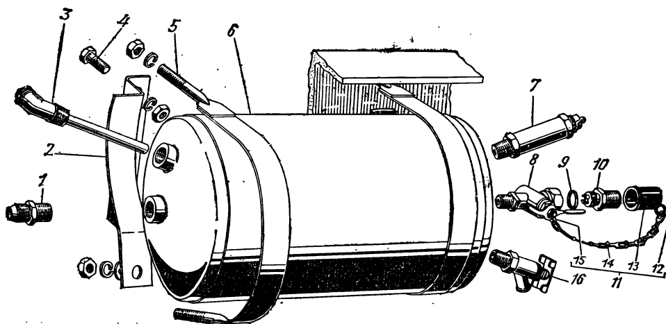
Рис 67. Воздушный баллон
