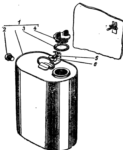
Рис. 64. Бачок для масла
