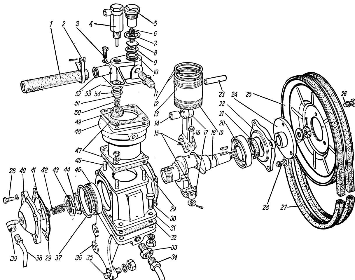
Рис. 65. Компрессор
