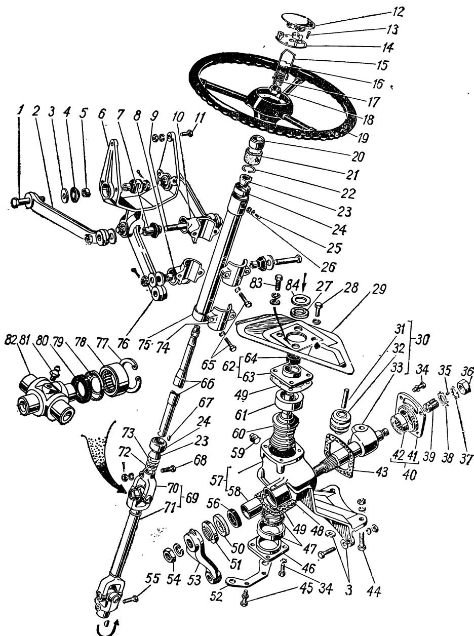
Рис. 42. Механизм рулевого управления
