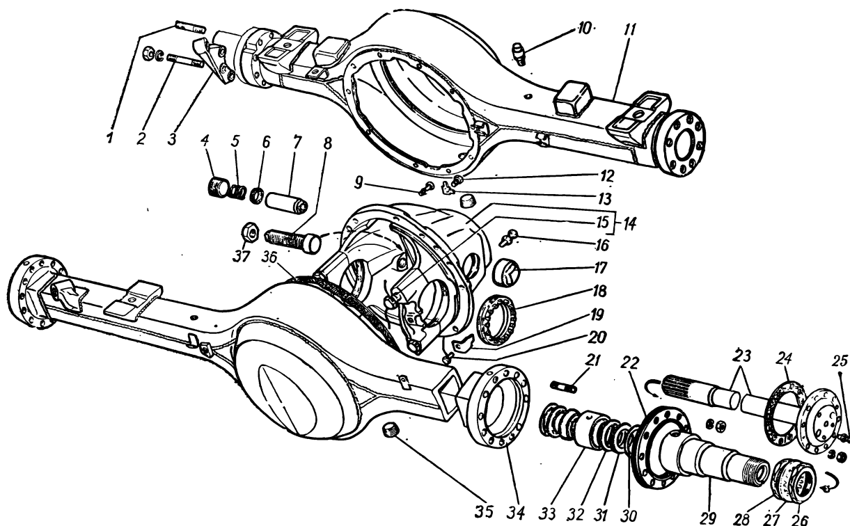
Рис. 31. Передний и задний мосты
