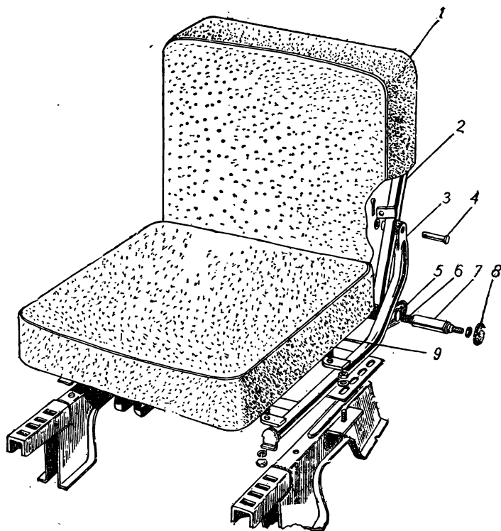
Рис. 80. Сиденье водителя
