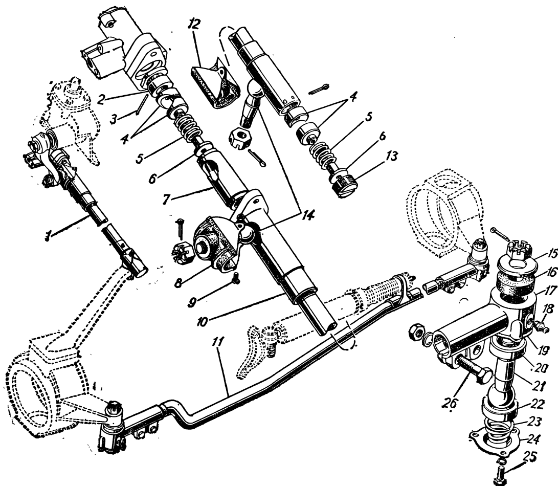
Рис. 39. Рулевые тяги
