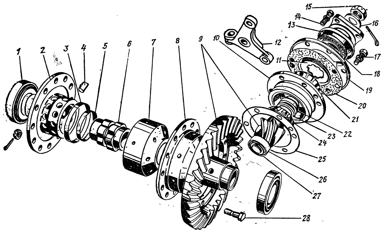
Рис. 32. Редуктор и дифференциал переднего и заднего мостов
