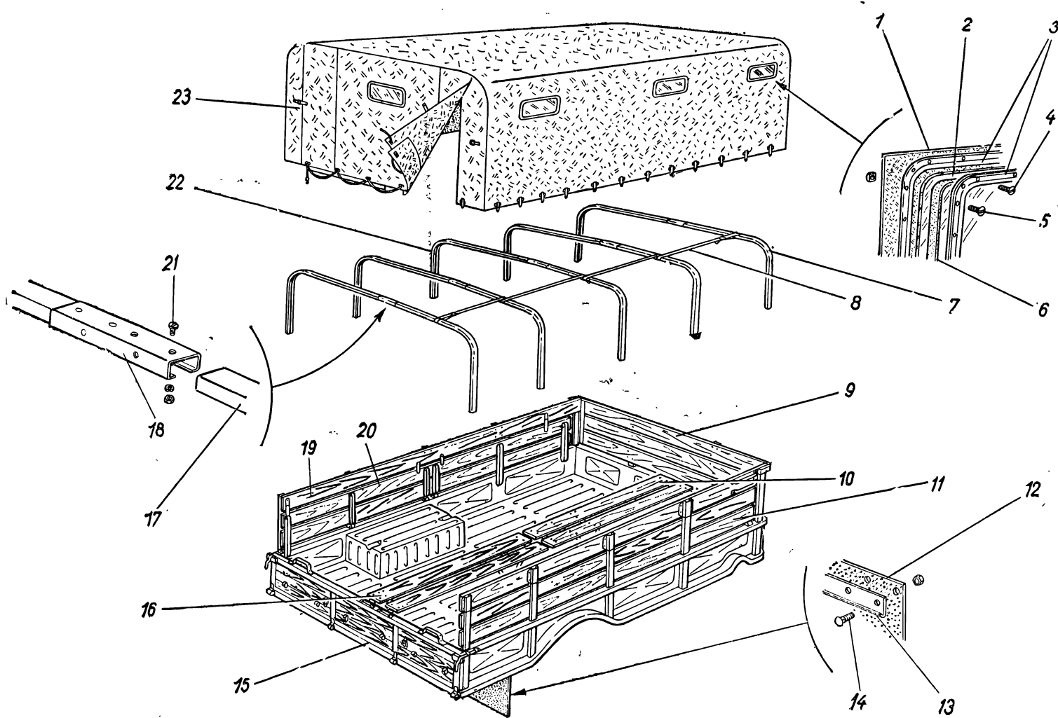
Рис. 83. Платформа
