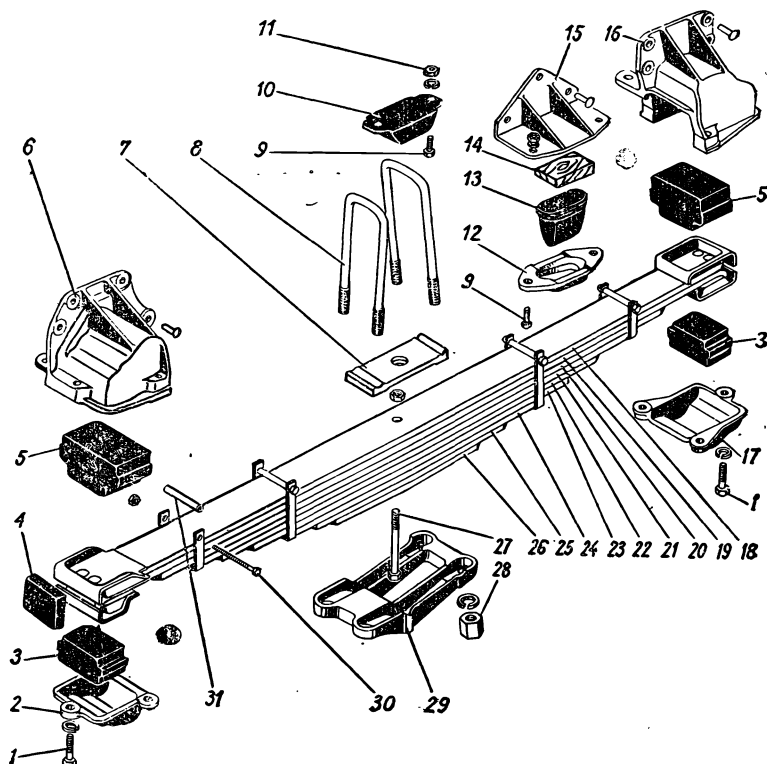
Рис. 37. Передние и задние рессоры
