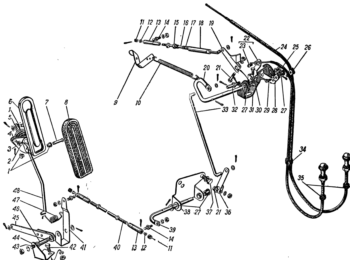
Рис. 17. Управление карбюратором
