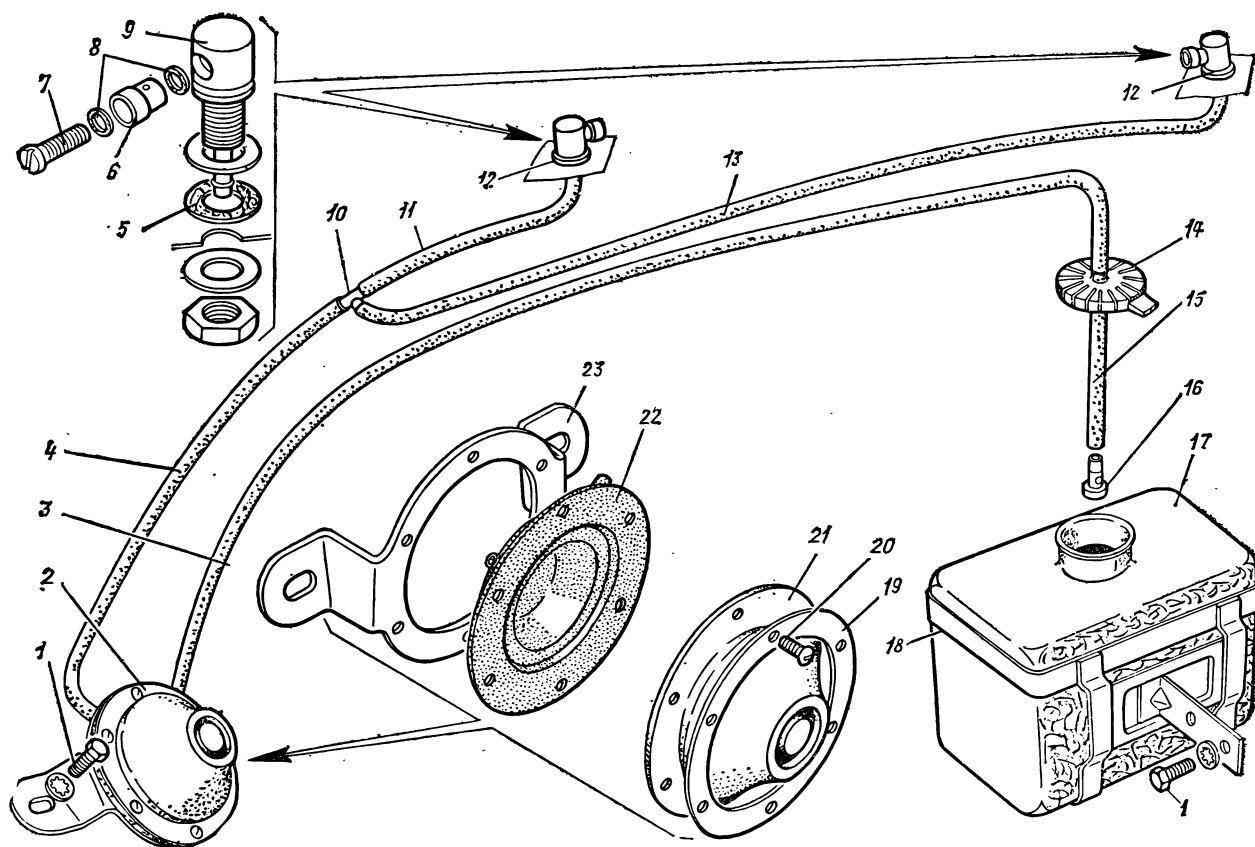
Рис. 76. Опрыскиватель ветрового стекла
