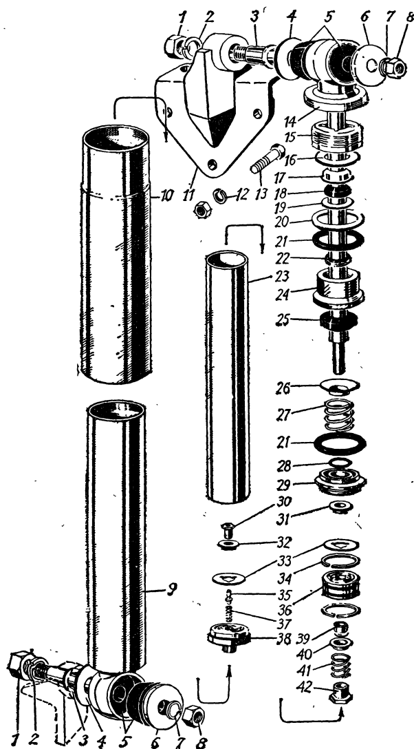
Рис. 38. Амортизаторы передней и задней подвесок
