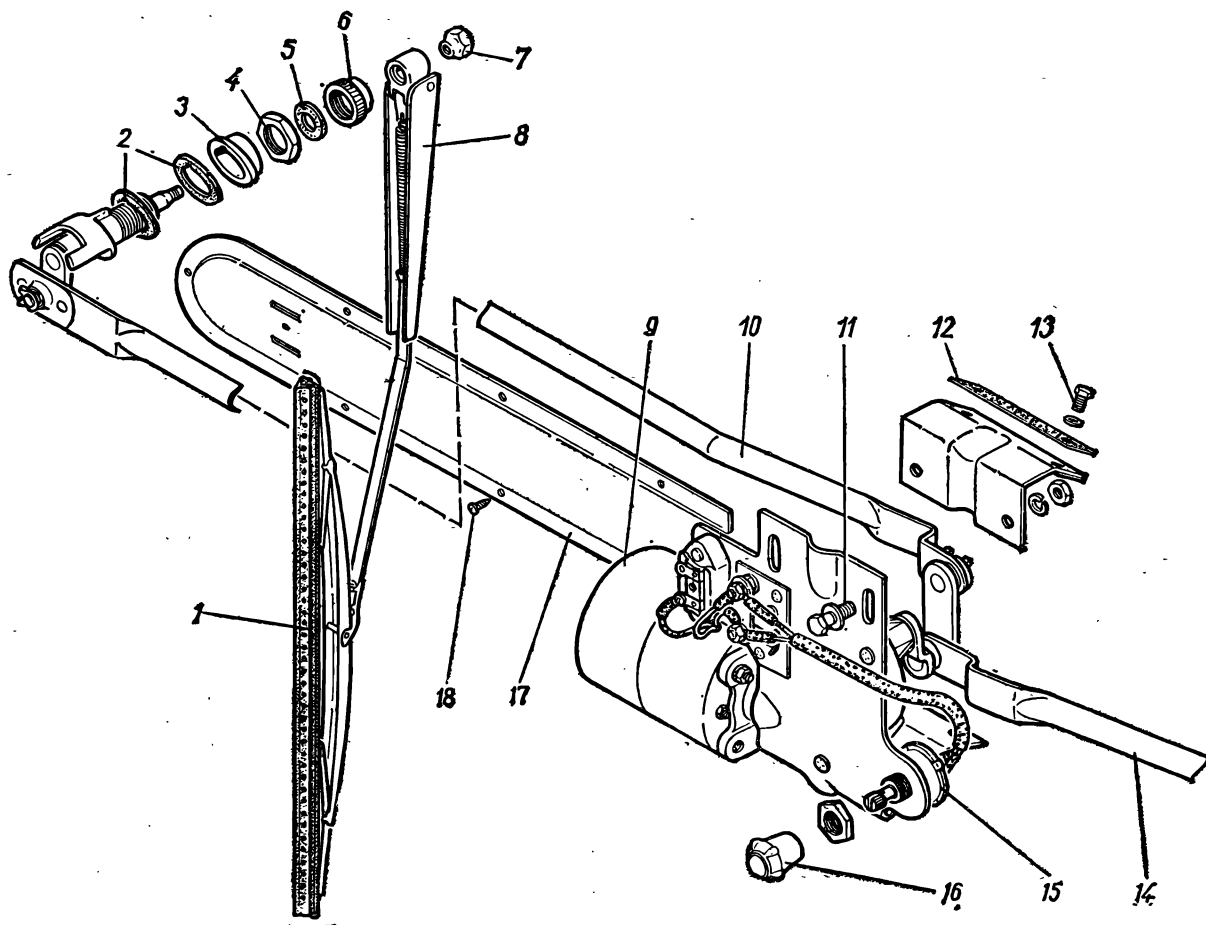
Рис. 75. Стеклоочиститель
