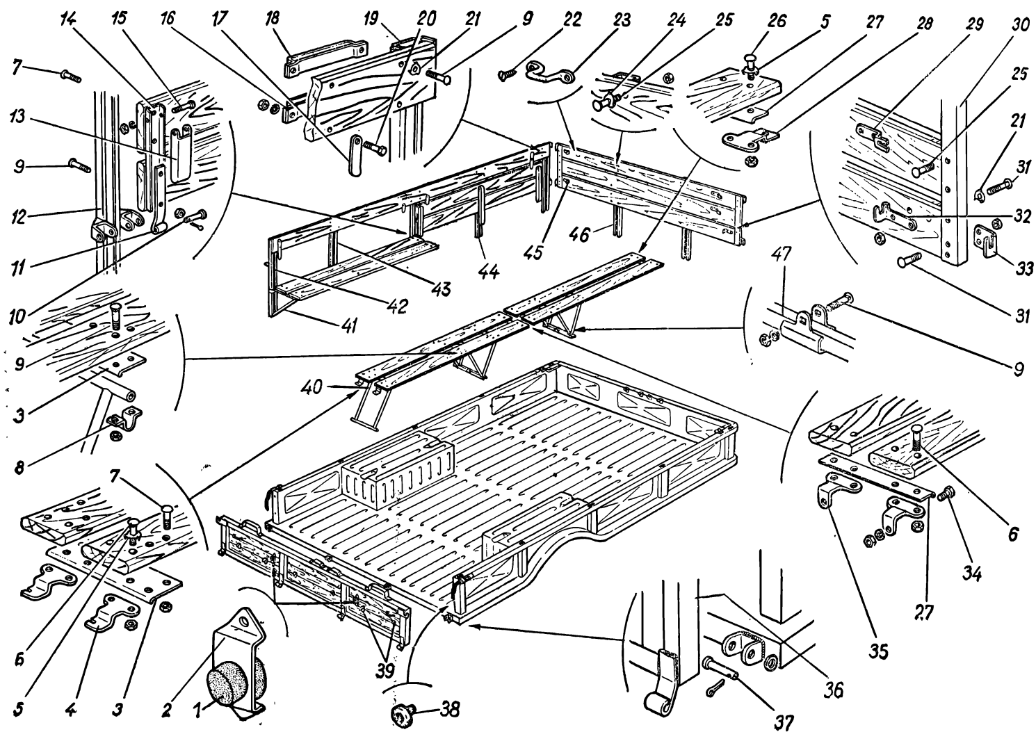
Рис. 84. Платформа
