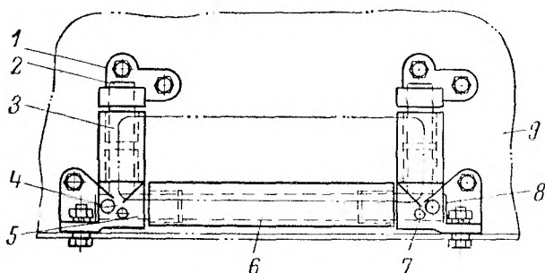
Рис. 113. Направляющее устройство троса лебедки; 1 и 5 — крошфейны; 2 — ось вертикальная; 3 и 6 — ролики; 4 — штифт; 7 — пресс-масленка; 8 — ось горизонтальная; 9 — бампер
