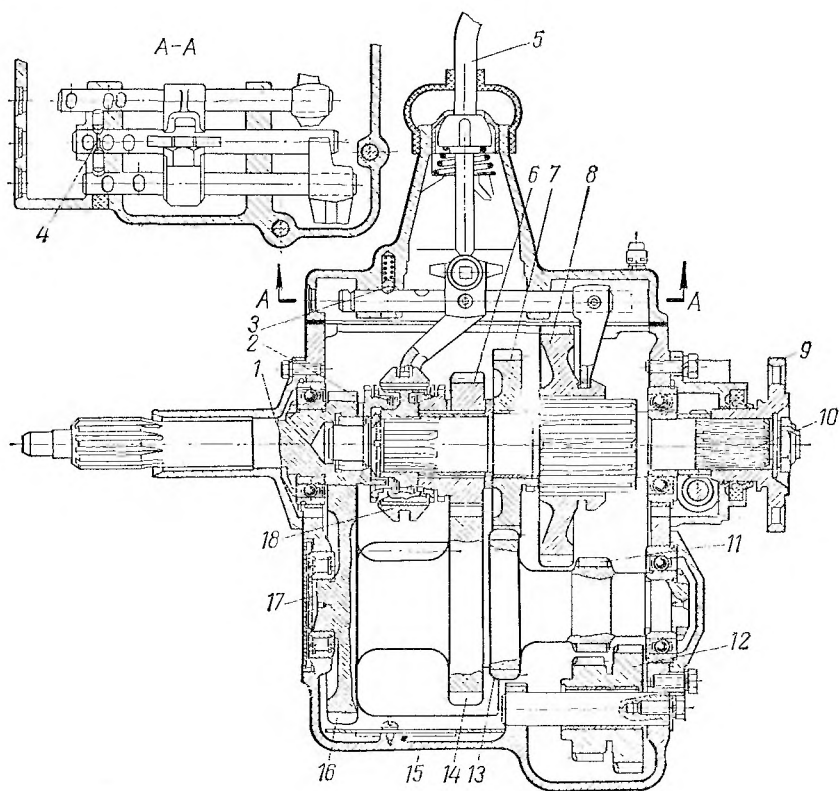
Рис. 38. Коробка передач:
