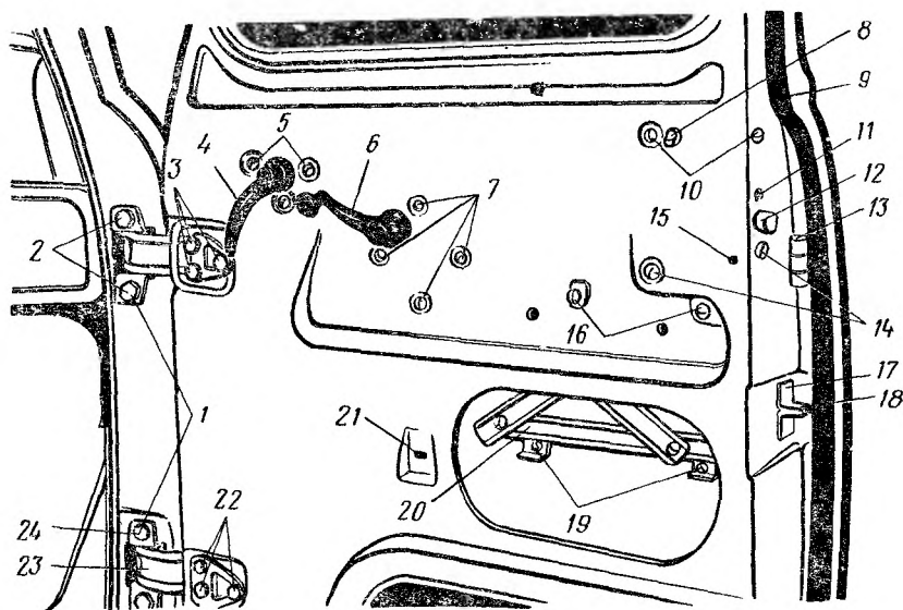
Рис. 158. Дверь кабины:
