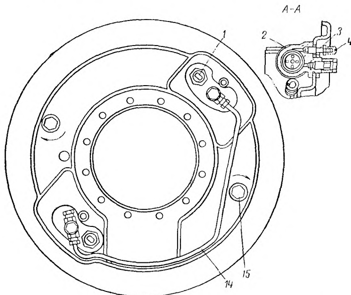
Рис. 99. Конструкция переднего
