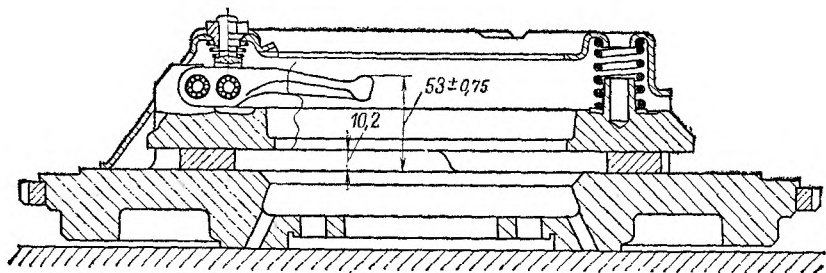
Рис. 35. Регулировка положения рычагов выключения сцепления
