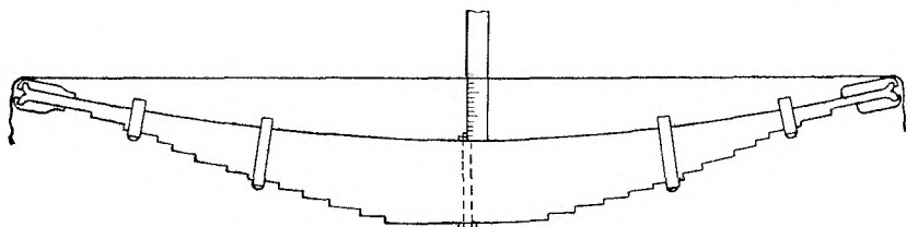
Рис. 79. Замер стрелы прогиба в свободном состоянии
