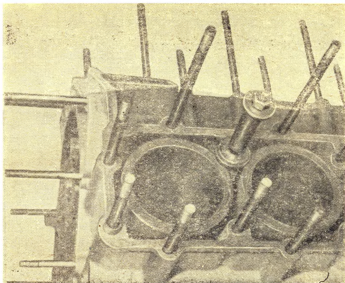
Рис. 13. Закрепление гильз в блоке цилиндров втулками-зажимами
