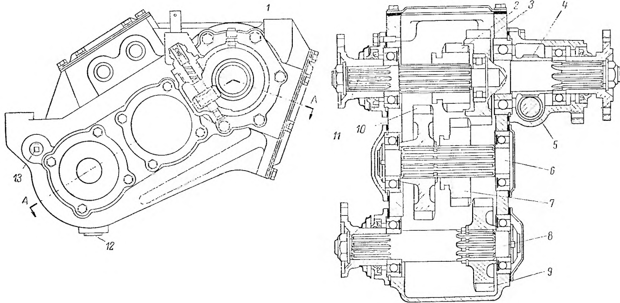
Рис. 50. Раздаточная коробка:
