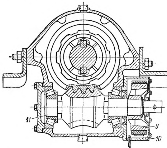
Рис. 108. Лебедка с редуктором: 1 — барабан; 2 — трос; 3 — муфта; 4 — рукоятка включения муфты барабана; 5 — пробка наливного отверстия; 6 — шестерня; 7 — картер; 8 — вал лебедки; 9 — автоматический тормоз; 10 — картер тормоза; 11 — червяк; 12 — сливная пробка
