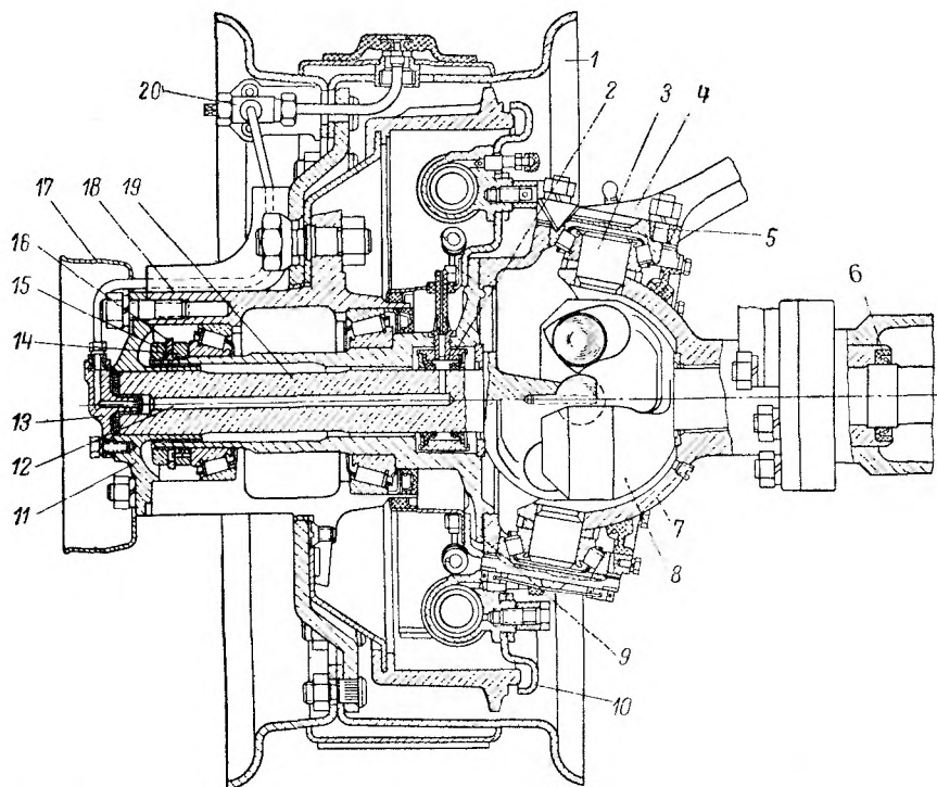
Рис. 74. Передний мост (привод к передним колесам автомобиля с системой регулирования давления воздуха в шинах):
