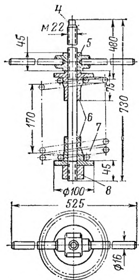
1 — стяжка двоякая наружная для правой пружины; 2 — стяжка внутренняя для правой пружины; 3 — стяжка левой пружины; 4 — винт приспособления; 5 — гайка верхняя; 6 — верхняя и нижняя опоры; 7 — пружина; 8 — опорная гайка
