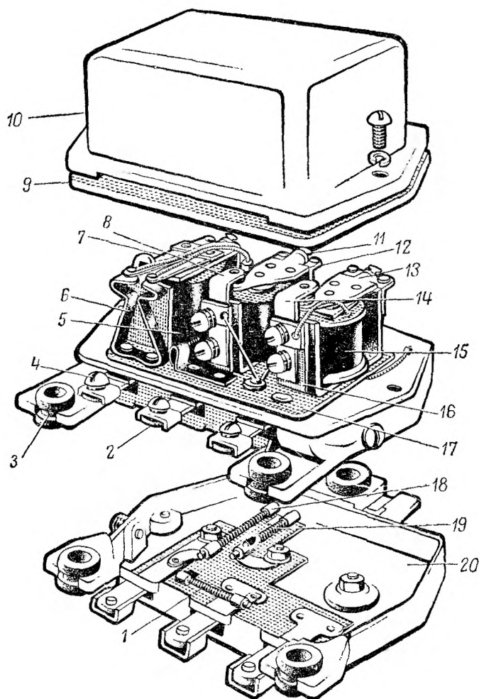
Рис. 131. Реле-регулятор PP130:
