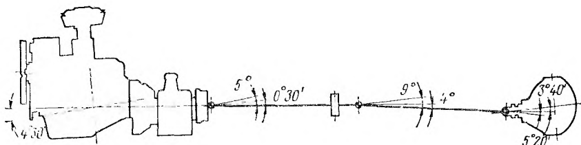
Рис. 57. Схема установки карданных валов автомобиля ГАЗ-53А
