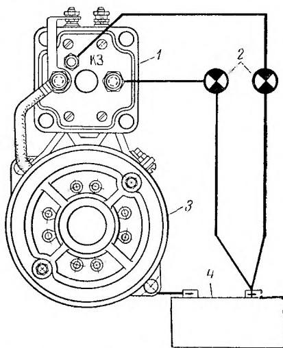
Рис. 139. Схема проверки регулятора включения стартера:
