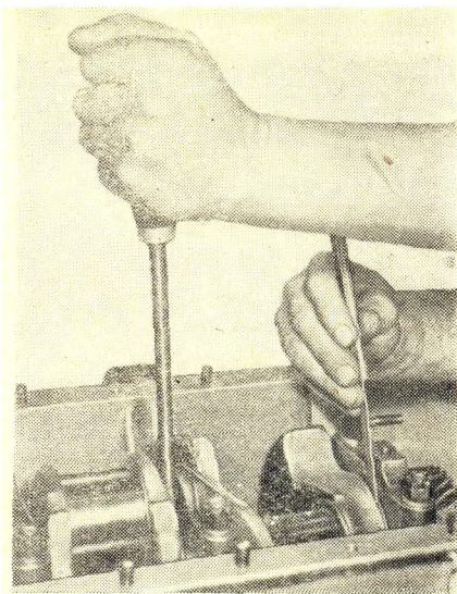
Рис. 26. Проверка осевого зазора
