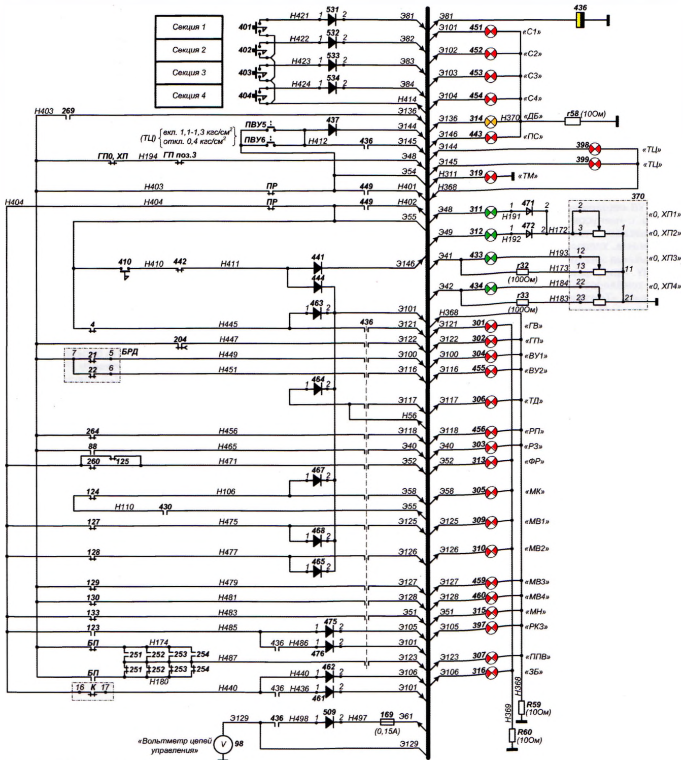
Схема цепей сигнализации электровоза ВЛ80С
