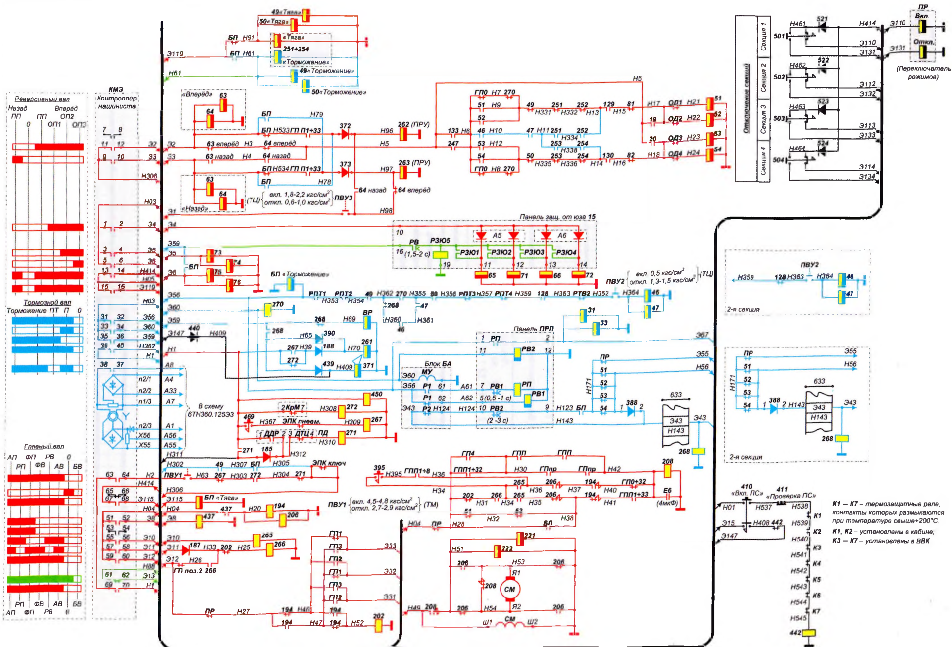
Схема цепей управления ТЭД электровоза ВЛ80С
