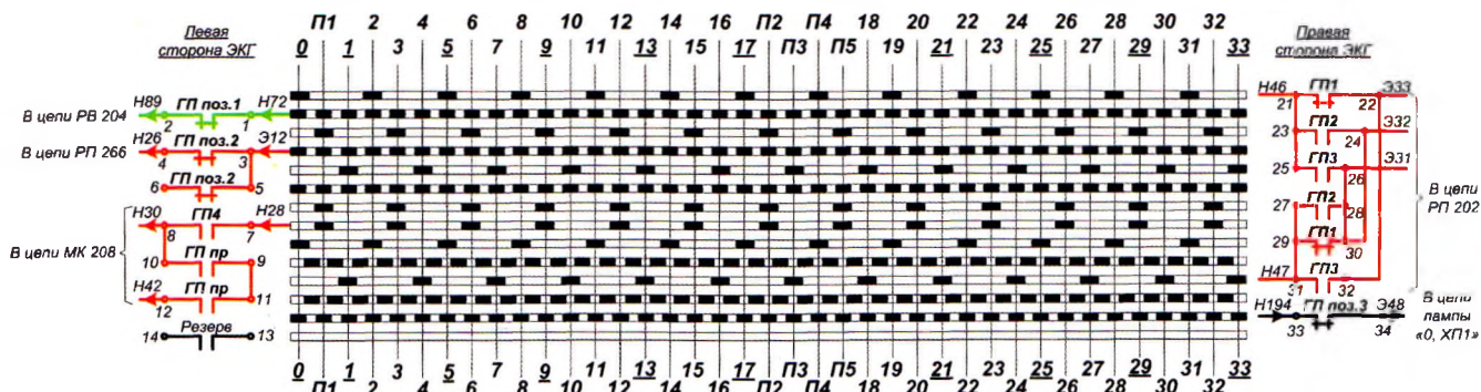
Диаграмма замыкания контактов верхнего блокировочного вала ЭКГ электровоза ВЛ80С
