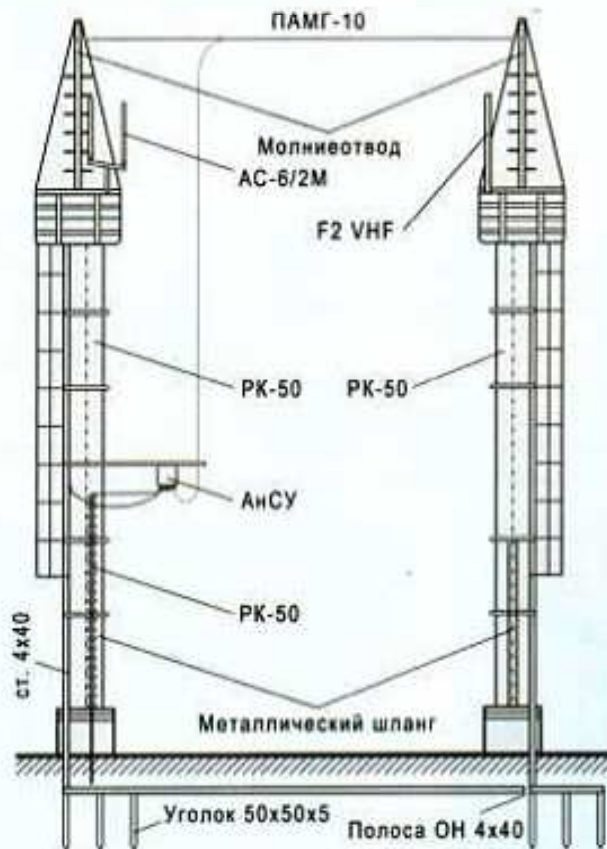
Конструкция Г-образной антенны, применяемой в Саратовской дирекции
