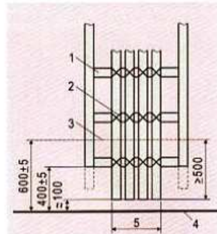
РИС. 3. Размещение образца на лестнице для испытаний в условиях воздействия пламени: 1 – круглые стальные перекладины; 2 – крепление металлической проволокой; 3 – центральная линия горелки; 4 – пол; 5 – максимальная ширина образца (в соответствии с категорией испытания)
