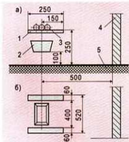
РИС. 2. Расположение образцов на опоре: А – вид сбоку; В – вид сверху; 1 – опора; 2 – металлический поддон; 3 – испытуемый образец; 4 – задняя стенка; 5 – пол
