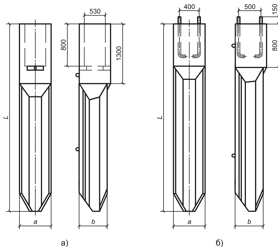
Рисунок 1 — Трехлучевые фундаменты:
