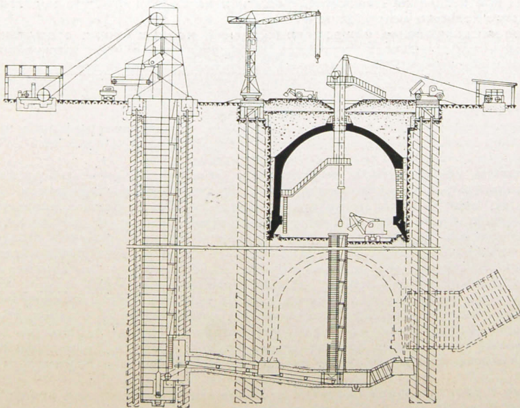
Схема опускания промежуточного вестибюля станции «Арсенальная».
