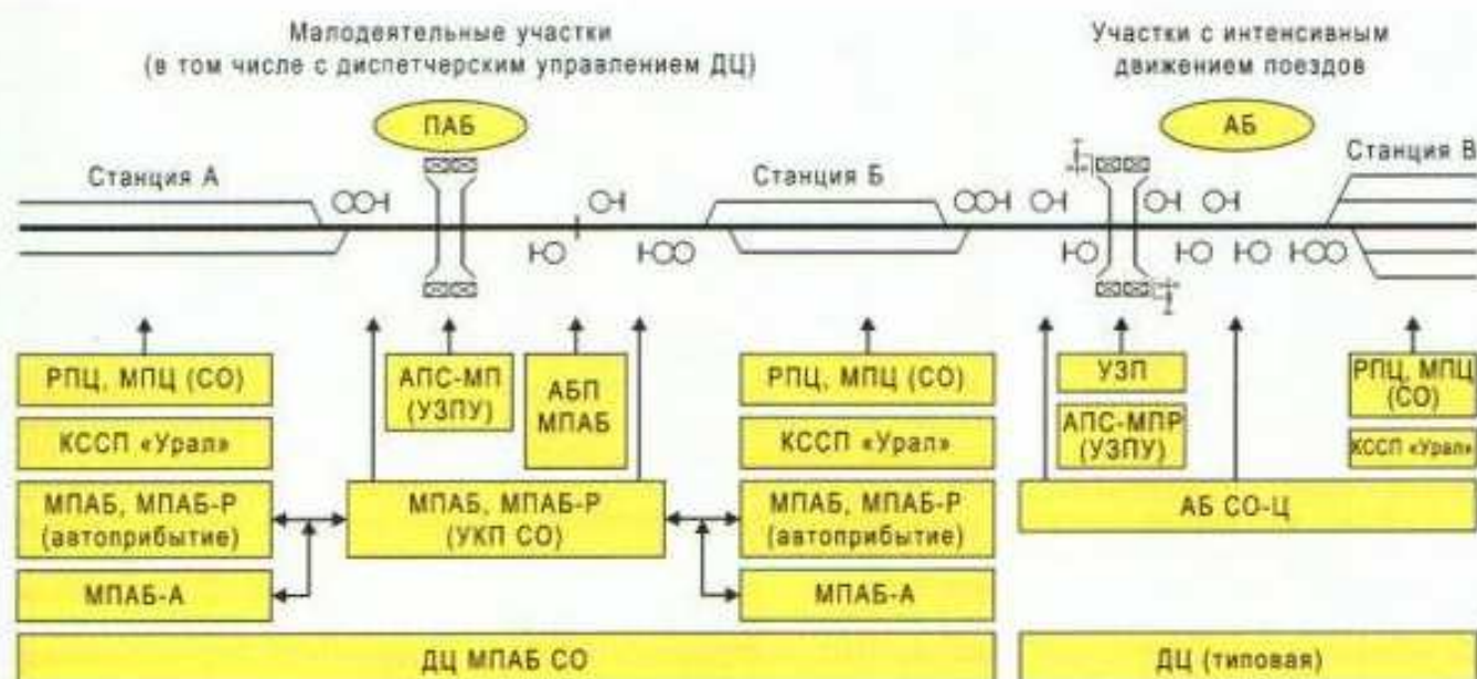
Комплексное оснащение участка железной дороги фирменными устройствами ЖАТ
