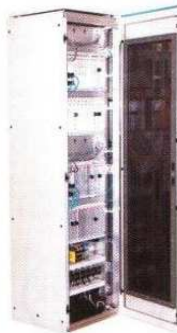
Типовой шкаф УБК
