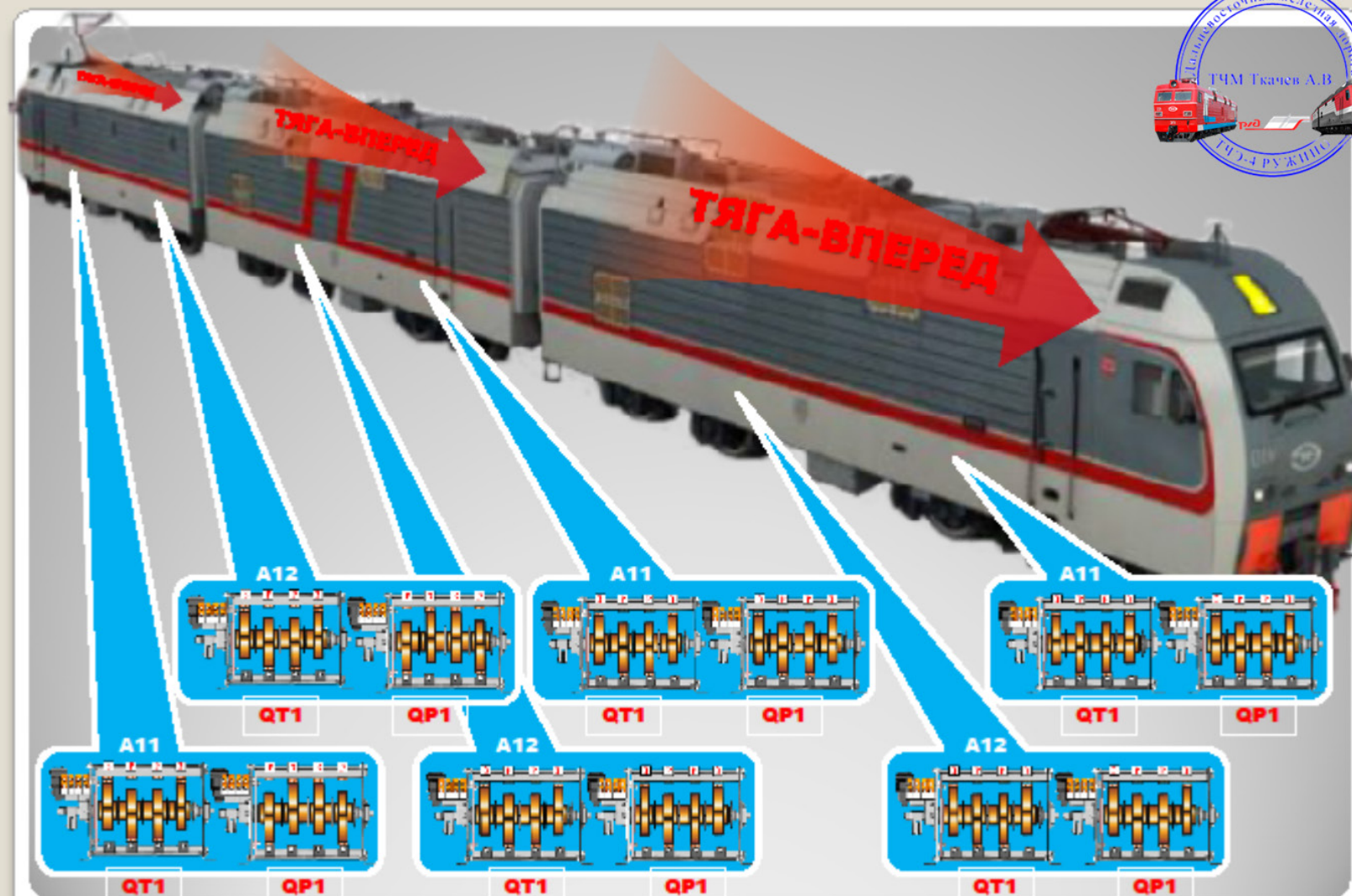
Положение QT1 QP1 в режиме ТЯГА направление ВПЕРЕД
