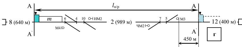
Рисунок 1.2 – Определение расчетной длины полурейса
