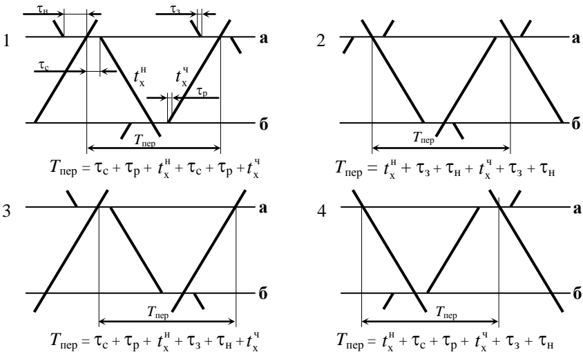
Рисунок 4.1 – Периоды парного непакетного графика движения поездов
