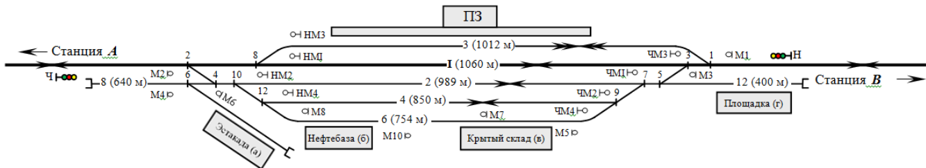
Рисунок 1.3 – Схема промежуточной станции к
