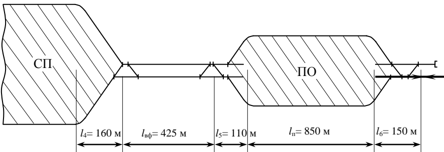
Рисунок 3.1 – Схема вытяжек формирования и прилегающих к ним подсистем
