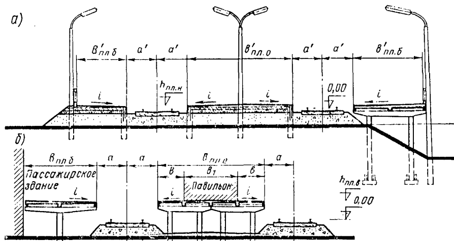
Рис. 6.1. Пассажирские железнодорожные платформы: а — низкие; б — высокие
