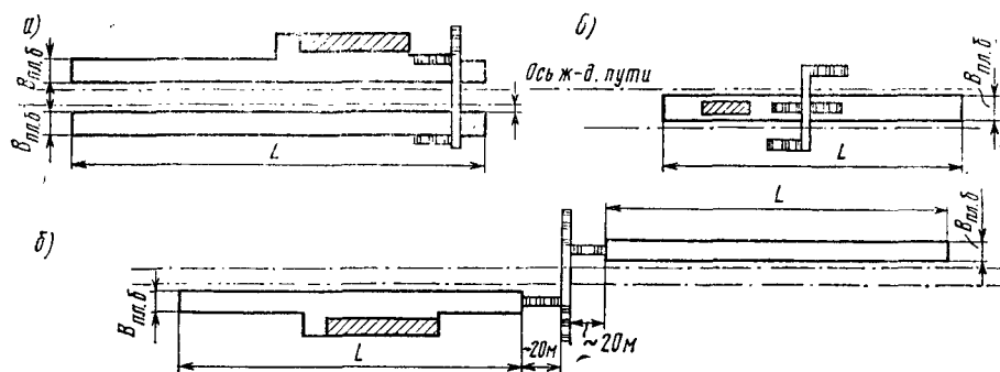
Рис. 6.2. Схемы размещения пассажирских платформ пригородных вокзалов на станциях сквозного типа:
