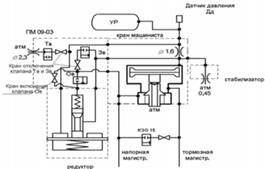
Рис. 1 Схема взаимодействия пневмомодуля с краном машиниста
