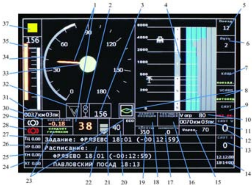
Рис. 4 Основной экран системы автоведения с блоком БС
