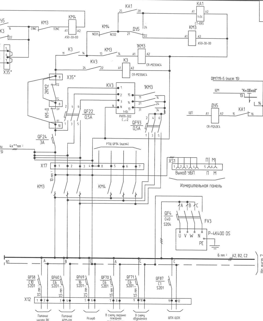
Распределительно-трансформаторный щит (РТЩ)
